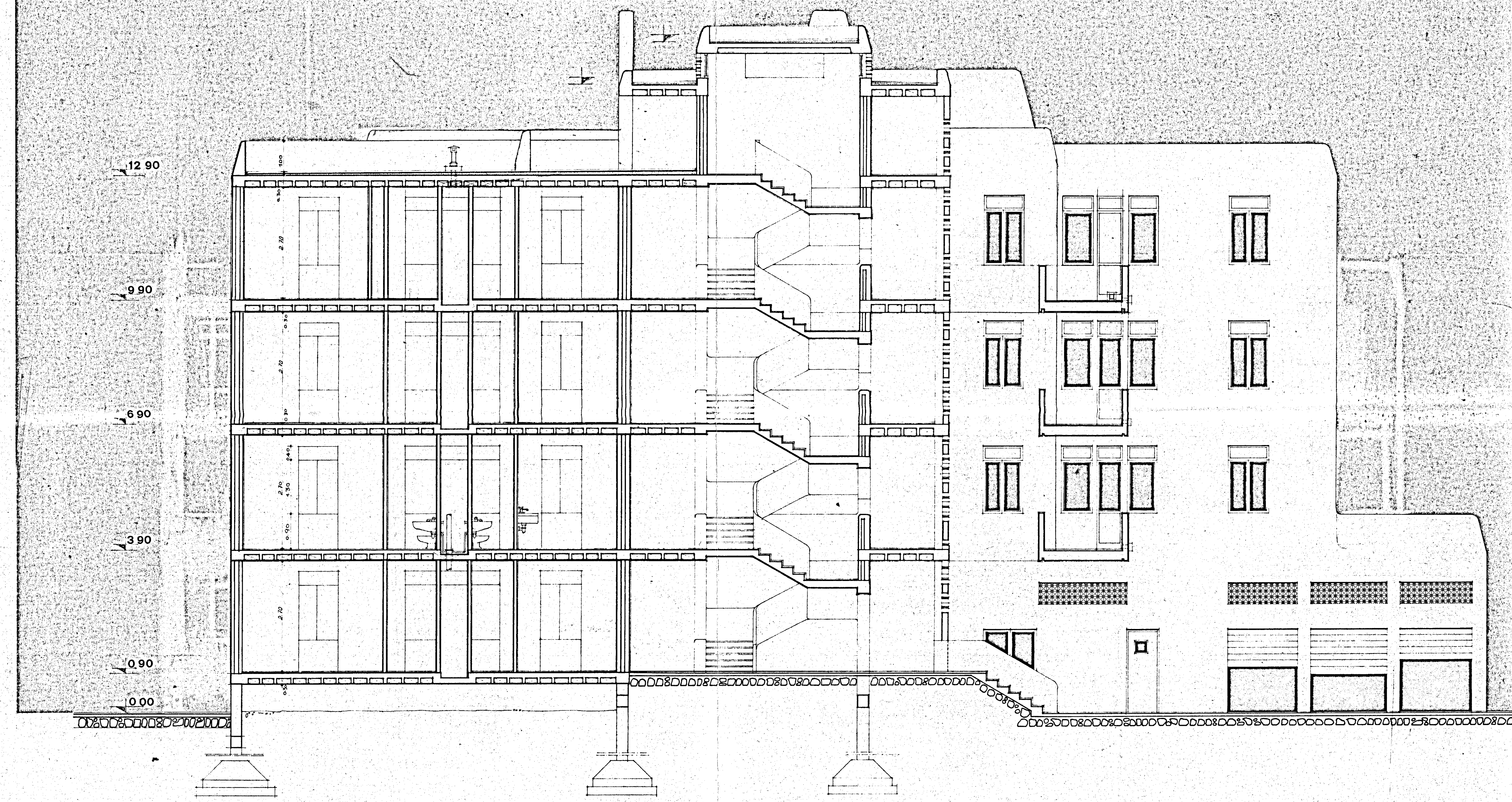
SEZIONE A-A'
