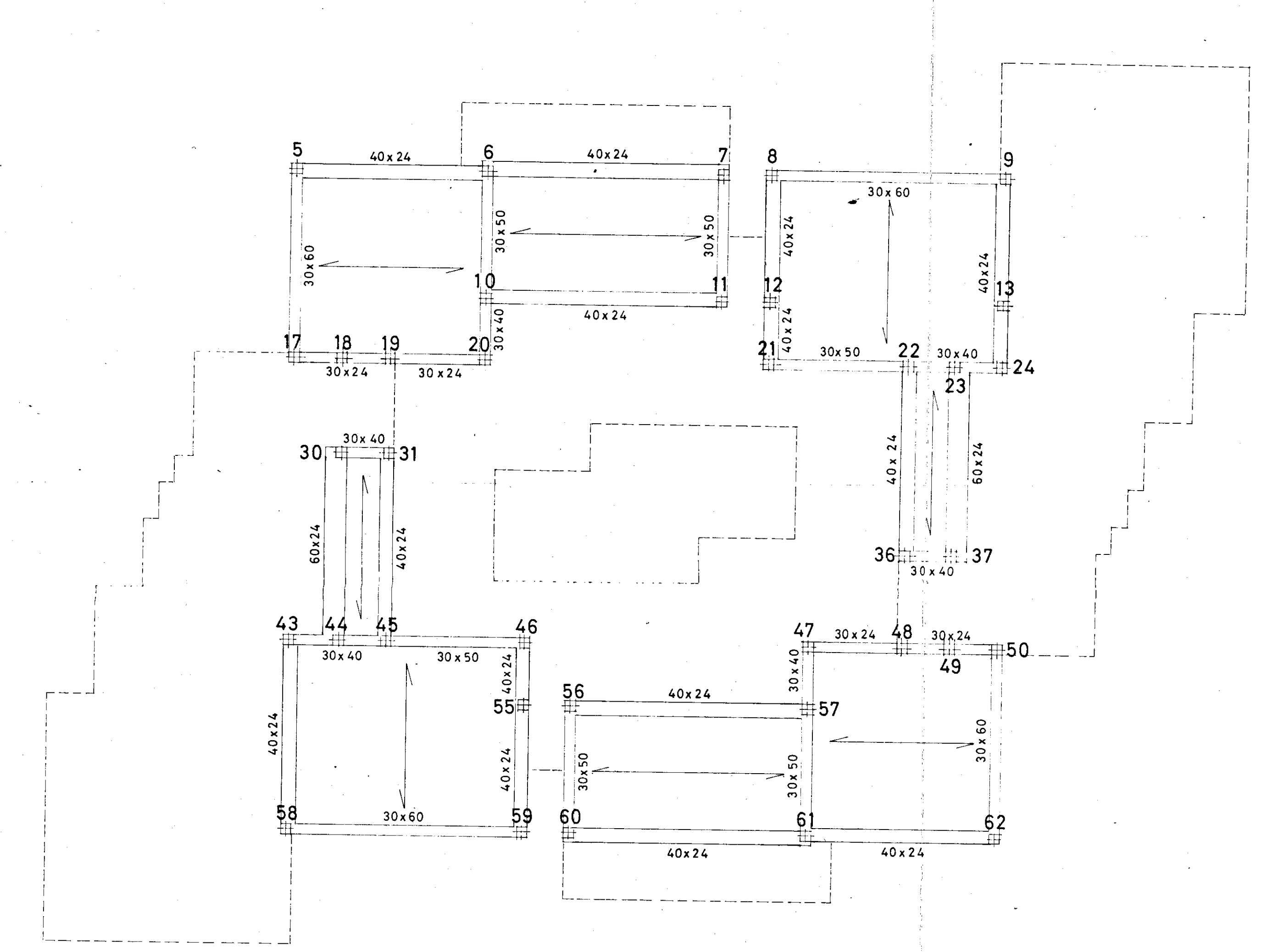
STRUTTURE A QUOTA +4,60
