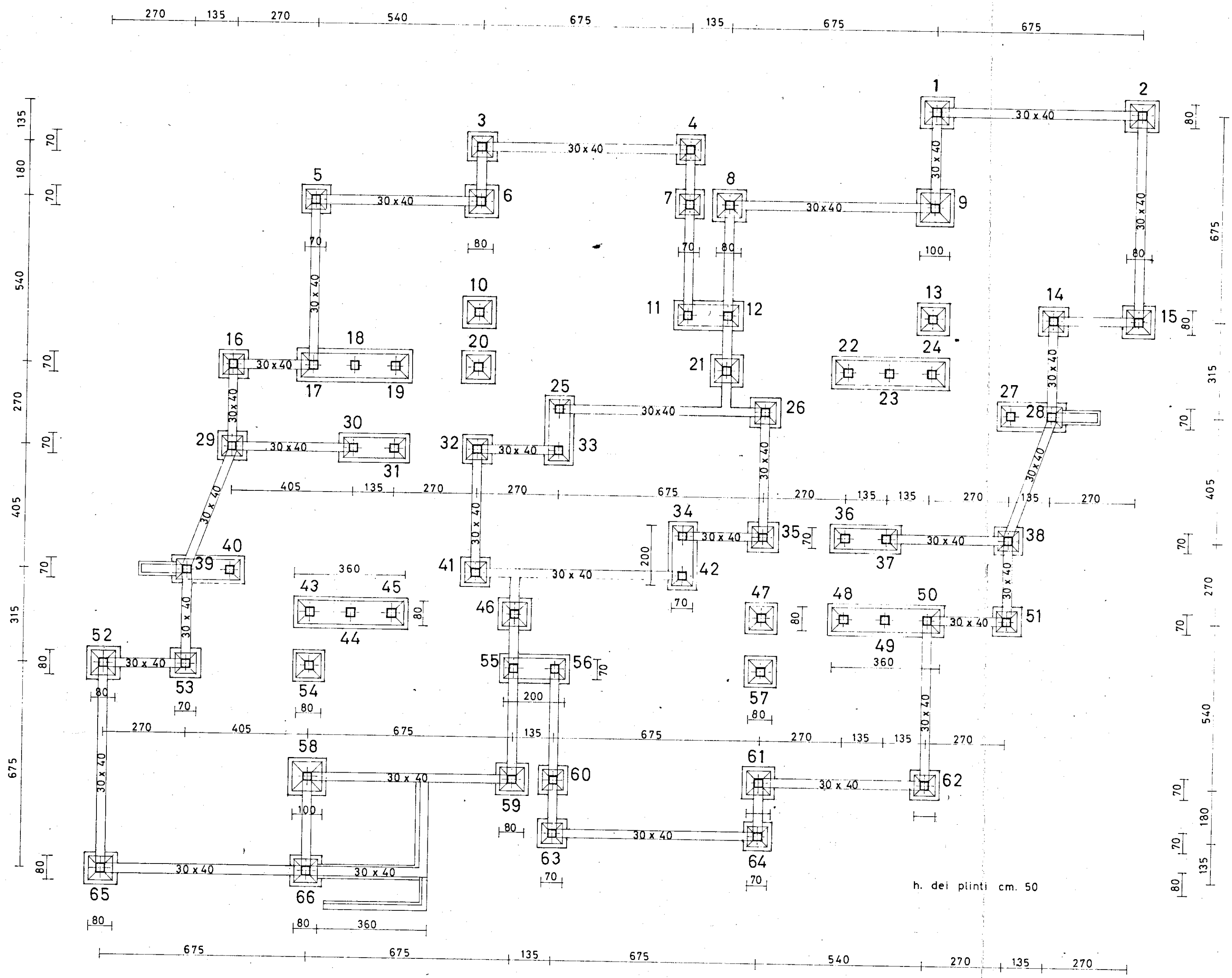
FONDAZIONI
