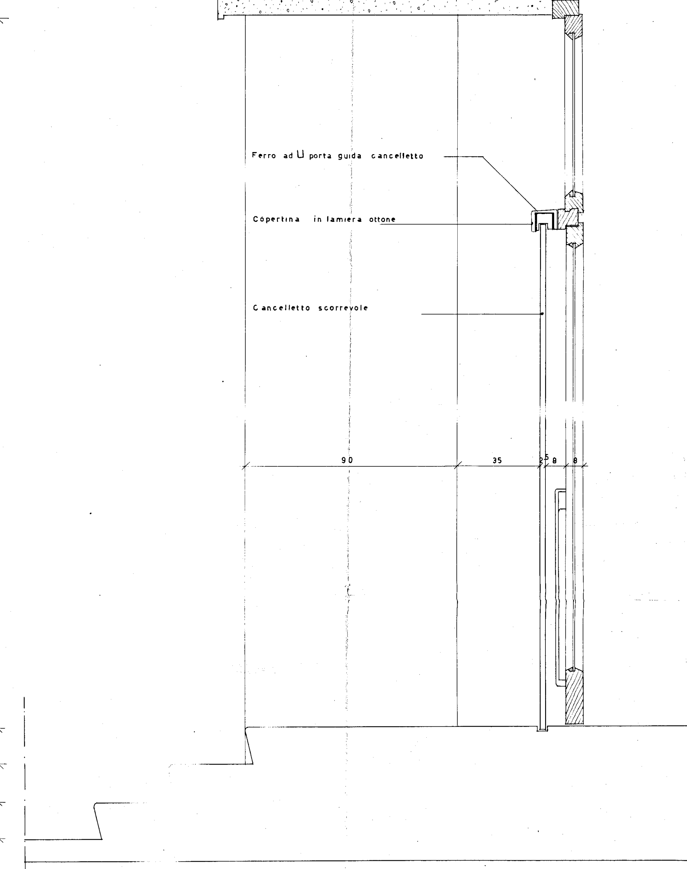
- SEZIONE A-B -
