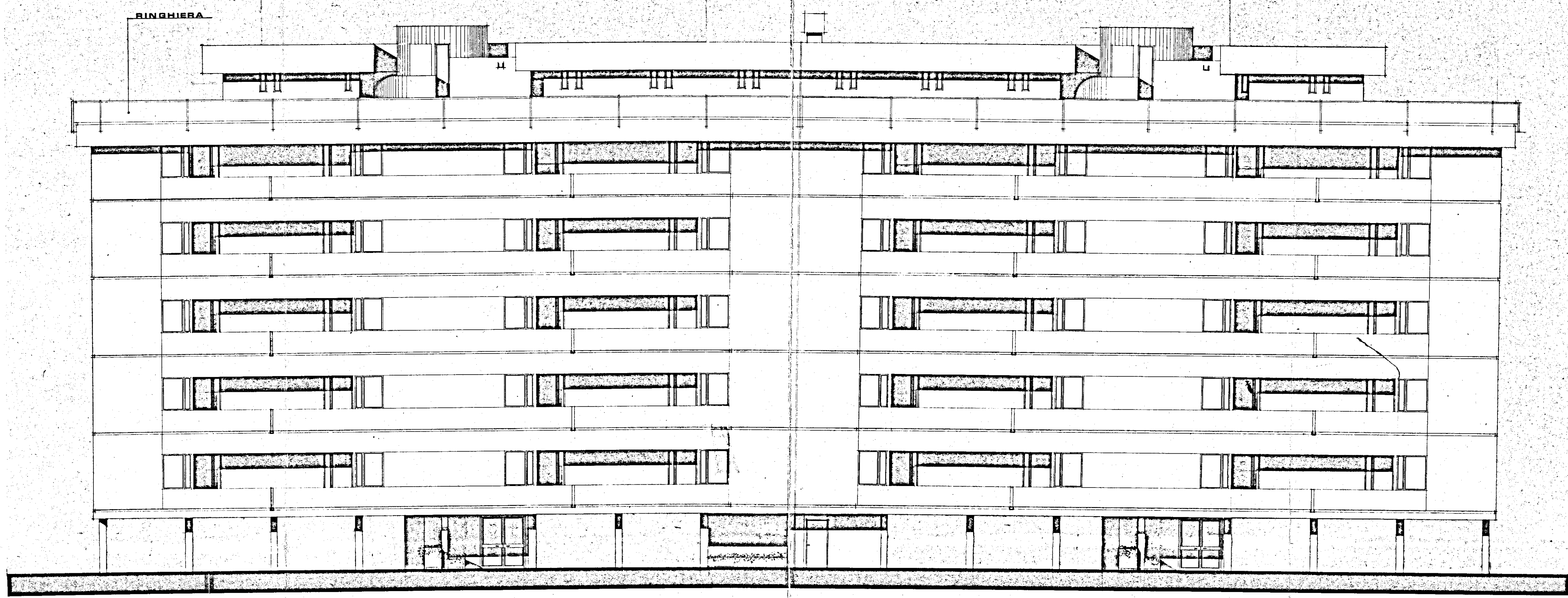
PROSPETTO EST
