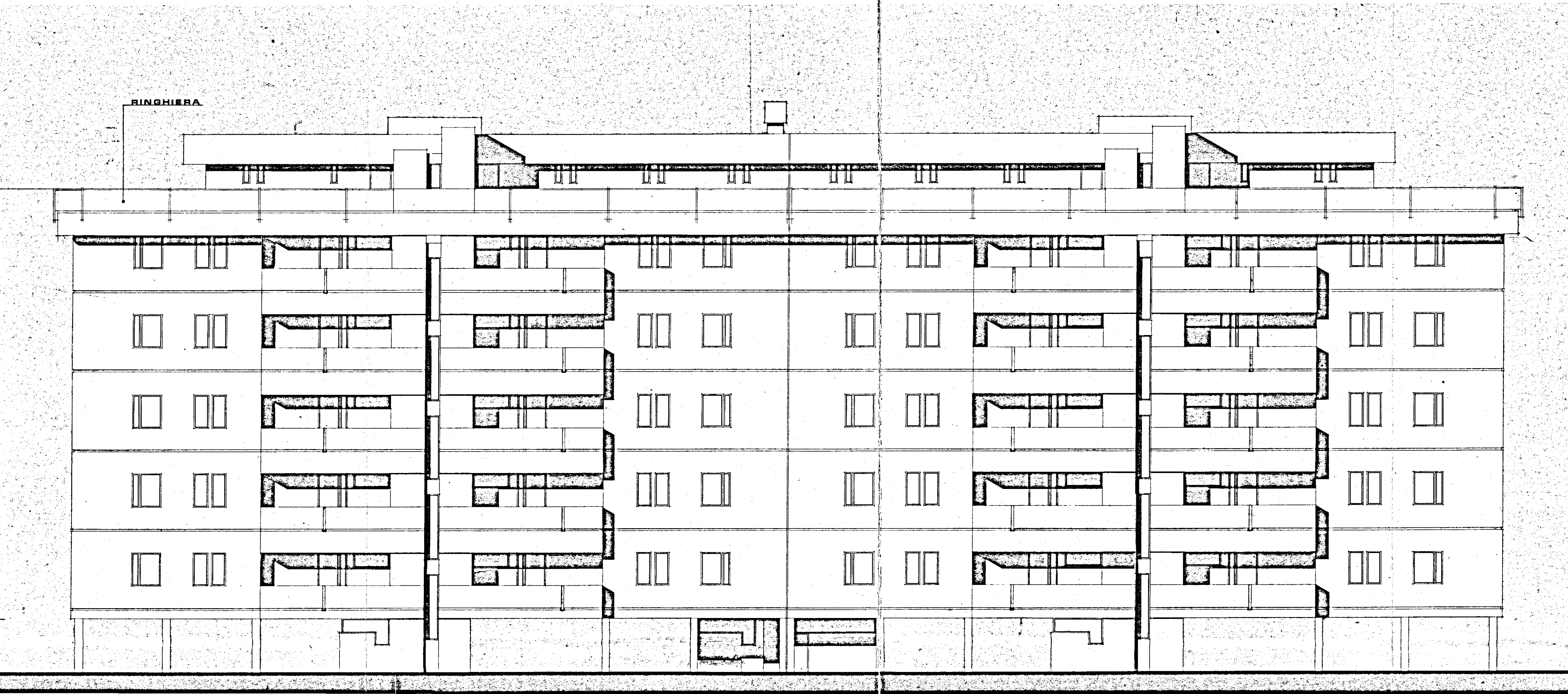
PROSPETTO OVEST
