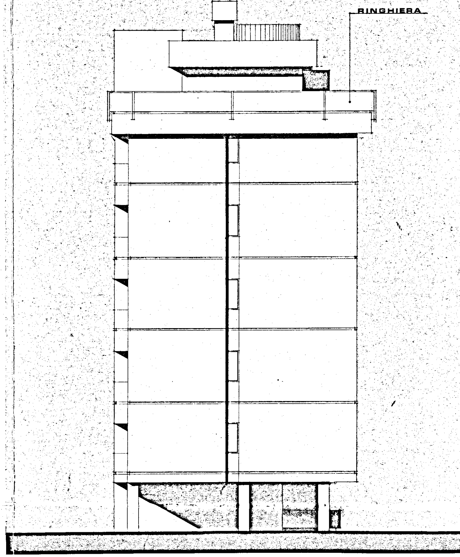
PROSPETTO SUD
