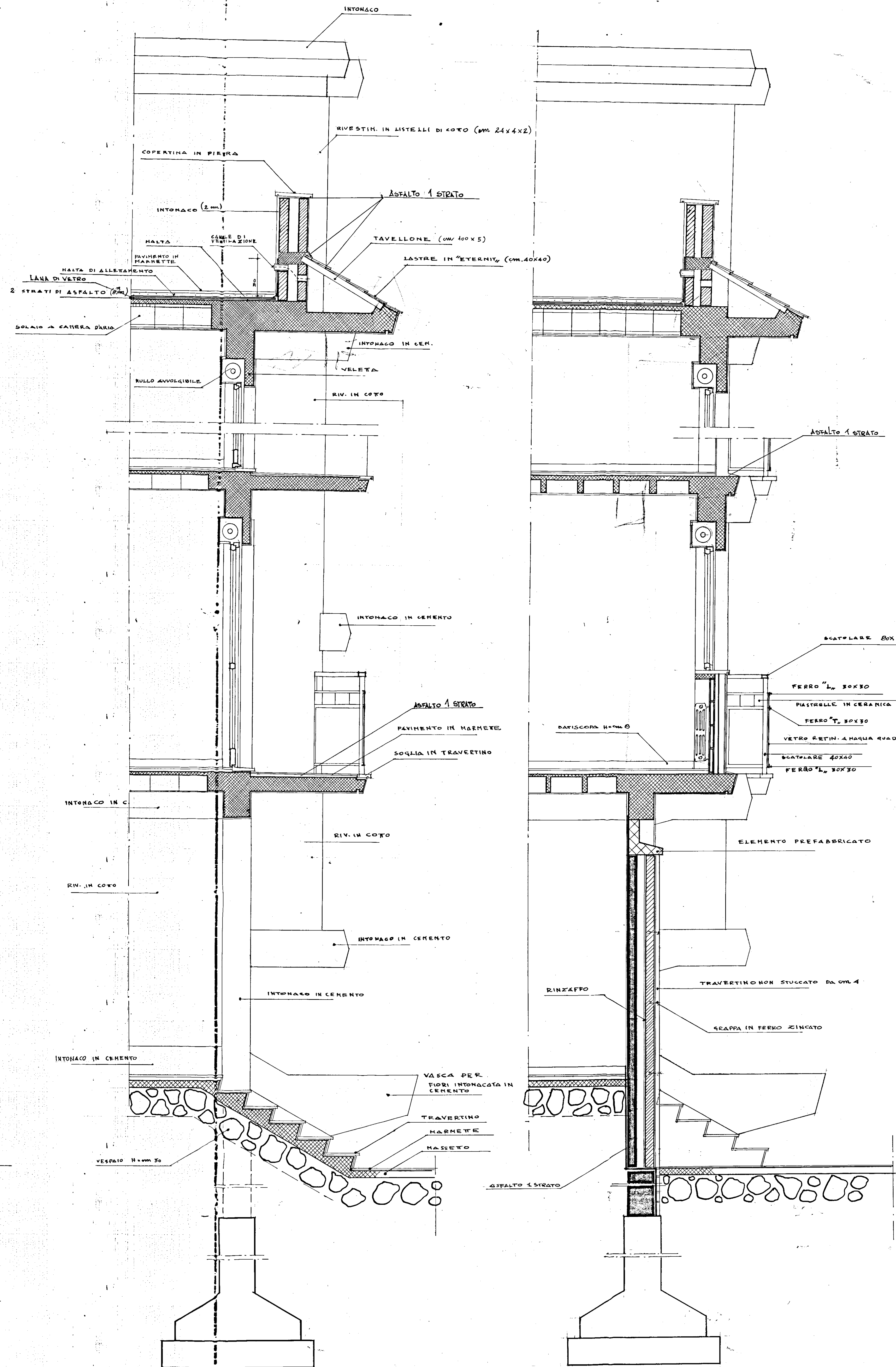
SEZIONE B-B
