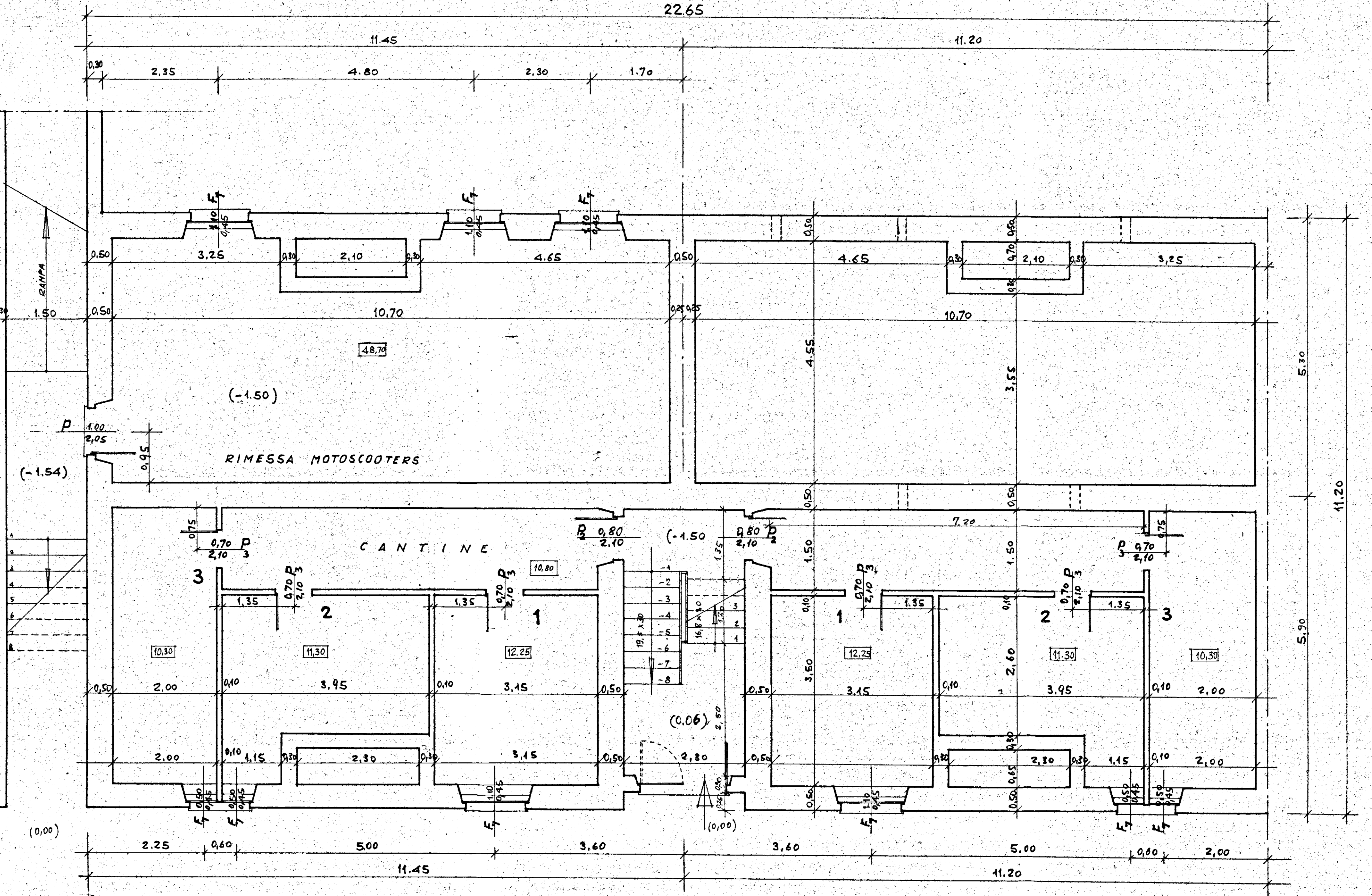
DIS. N° 166 bis PIANTA PIANO CANTINE E RIMESSA MOTO (PARTICOLARE DELLA PIANTA 159 bis) RAPP. 1:50
