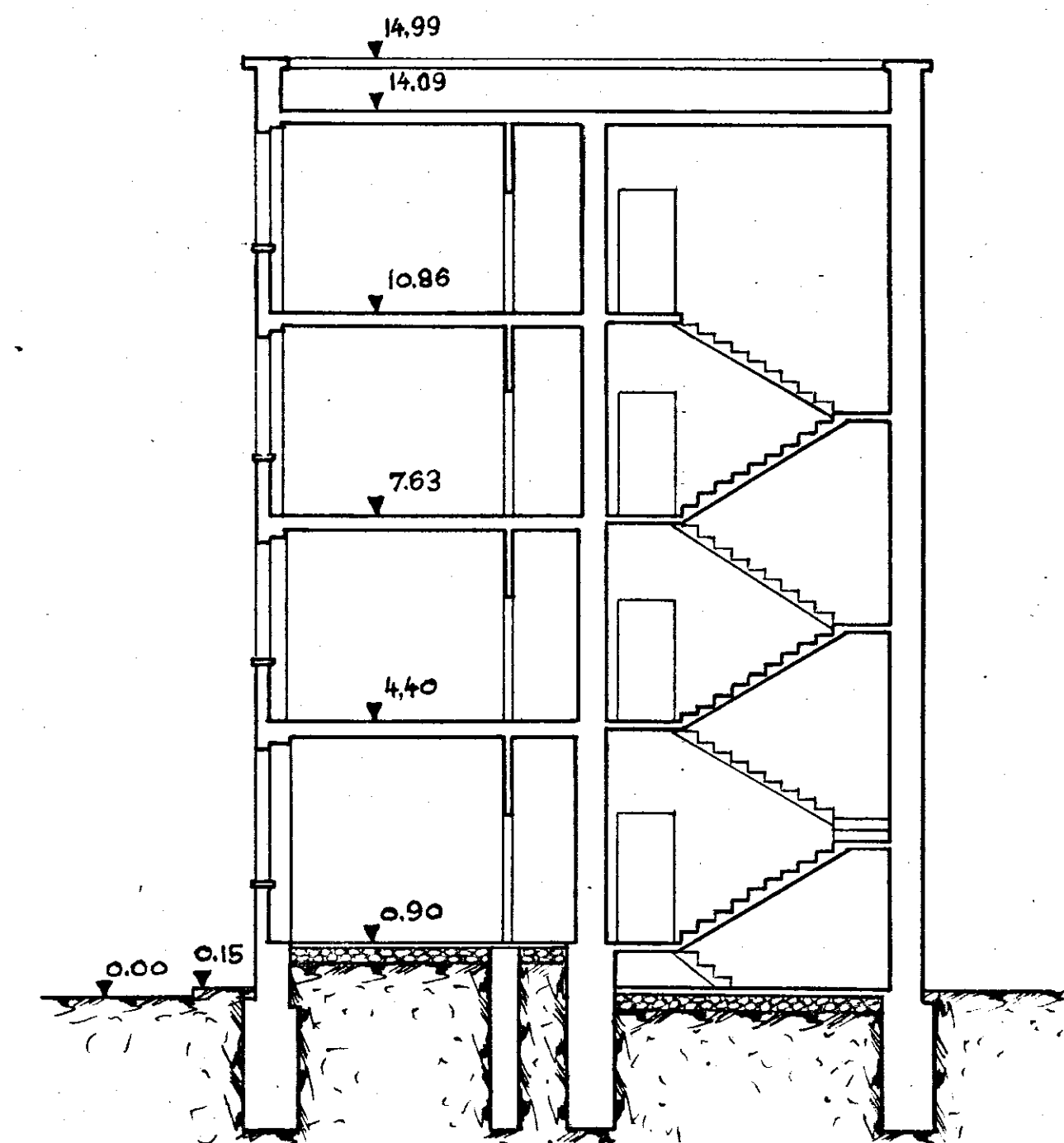
SEZIONE C-D
