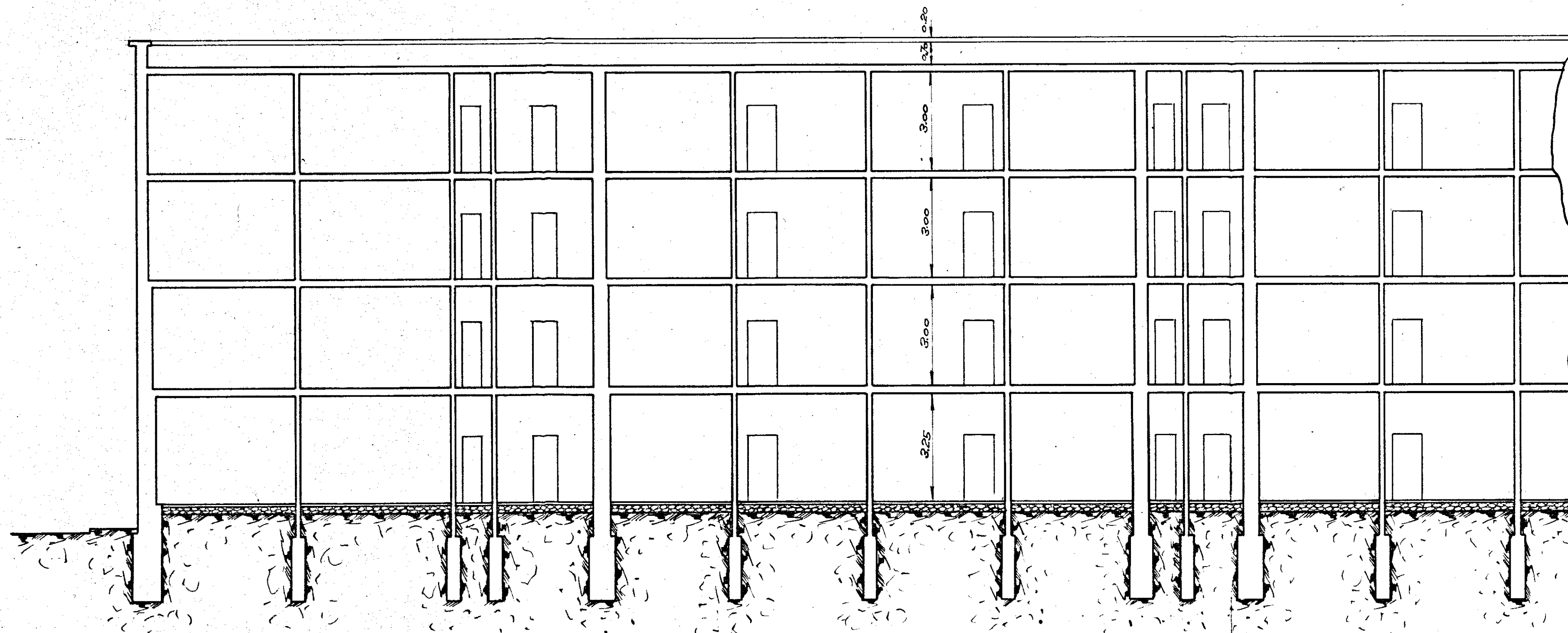
SEZIONE A-B
