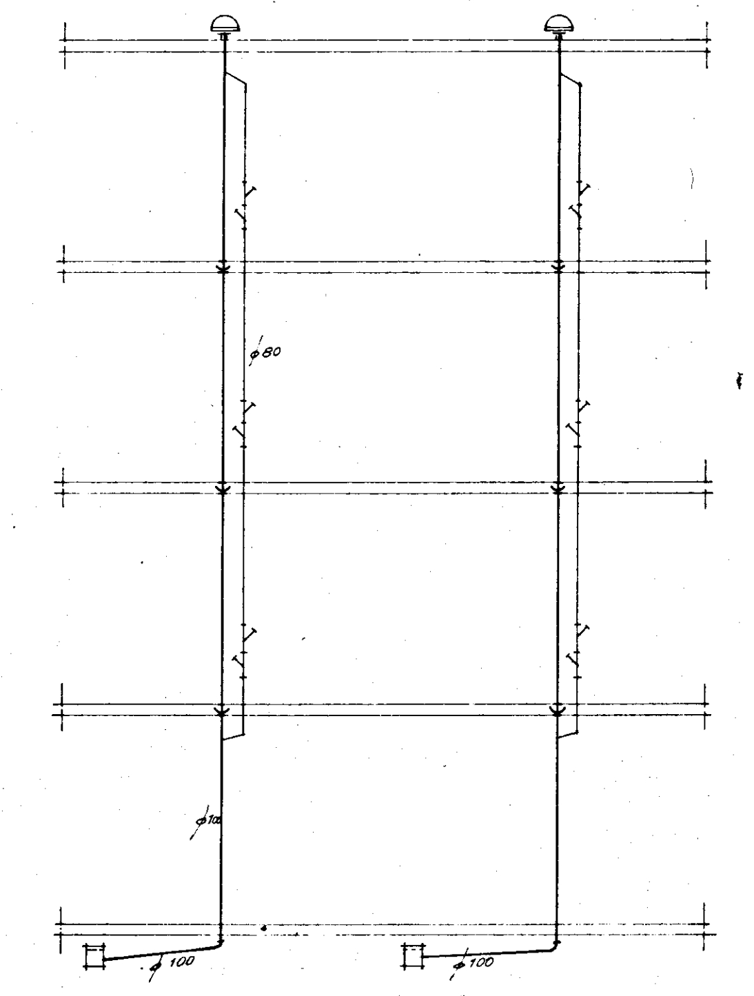
SCHEMA IMPIANTO POCNANTE Lotti 29-30
