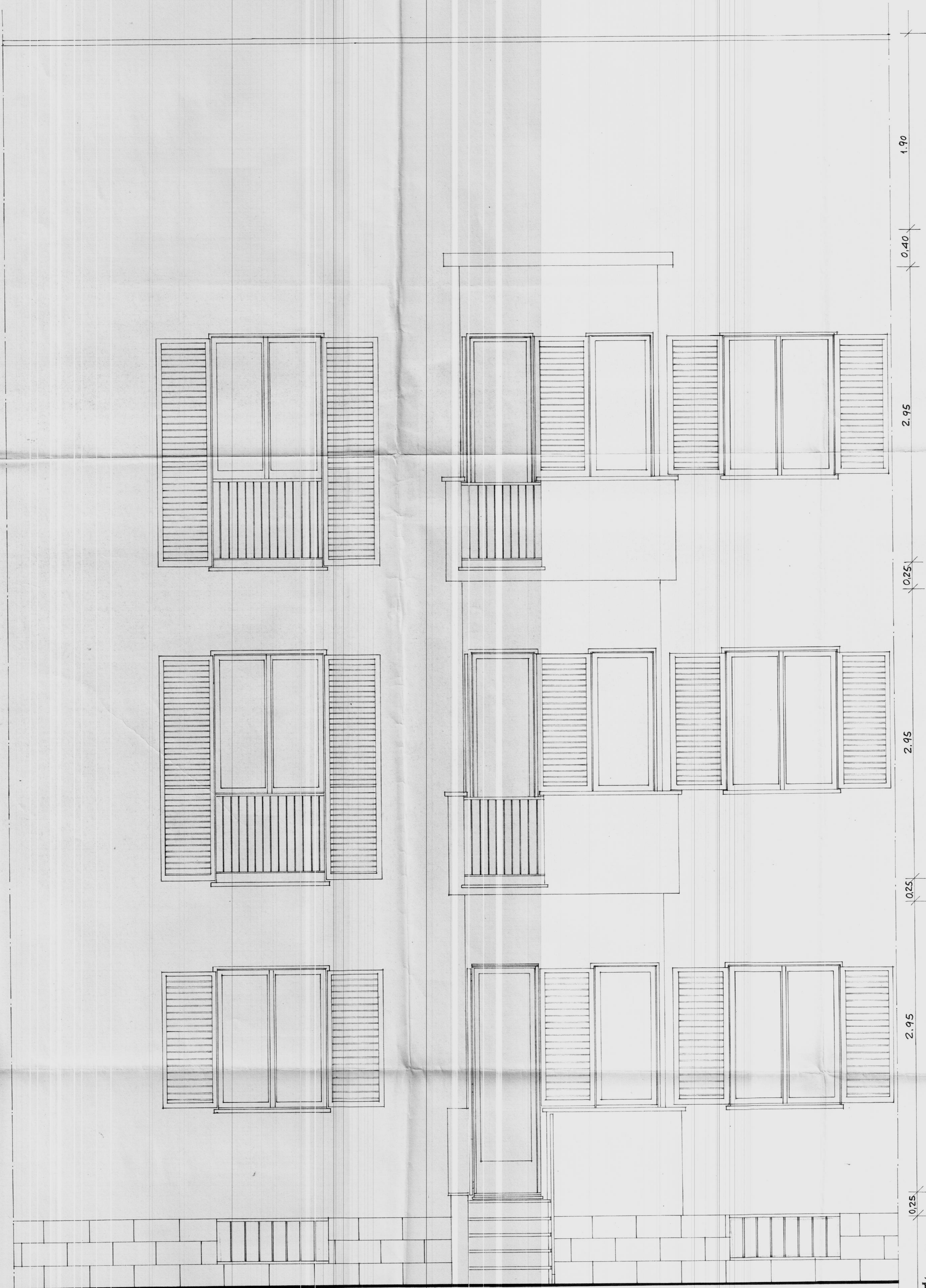
DIS. N° 237 PARTICOLARE DEL PROSPETTO A TAV. 29 DIS. N° 80
