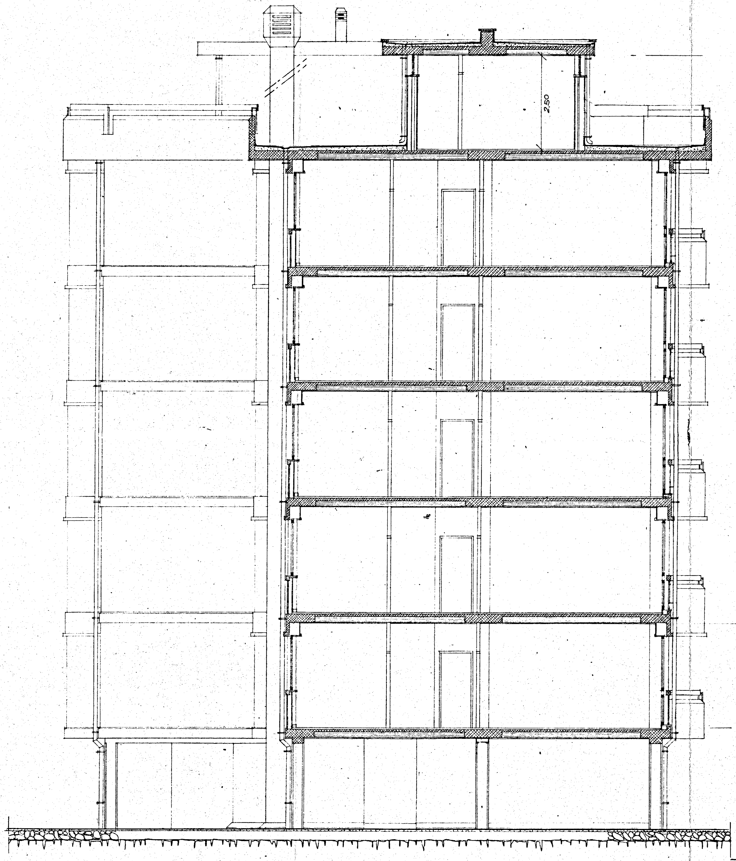
SEZIONE X-X
