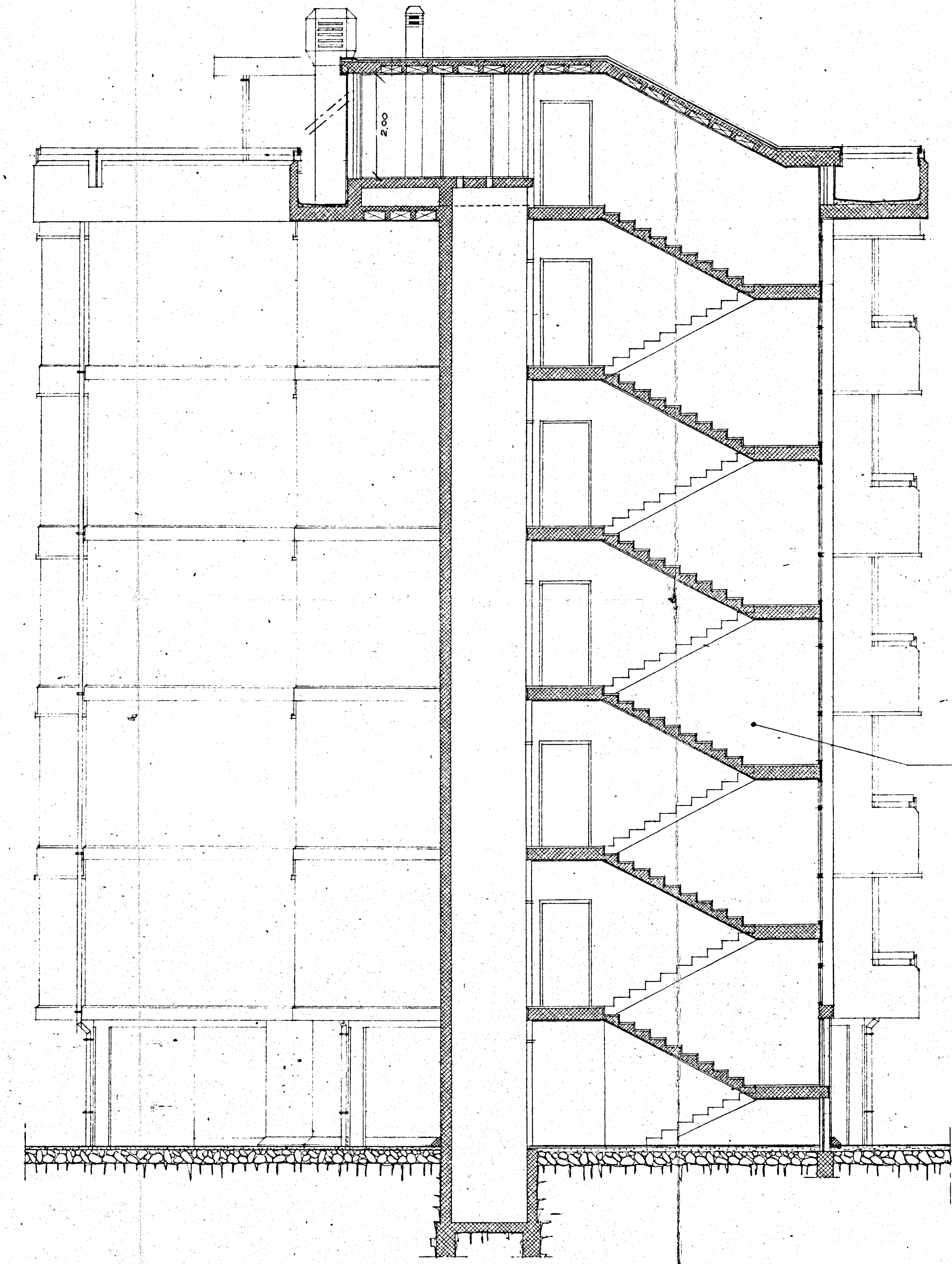
SEZIONE Y-Y
