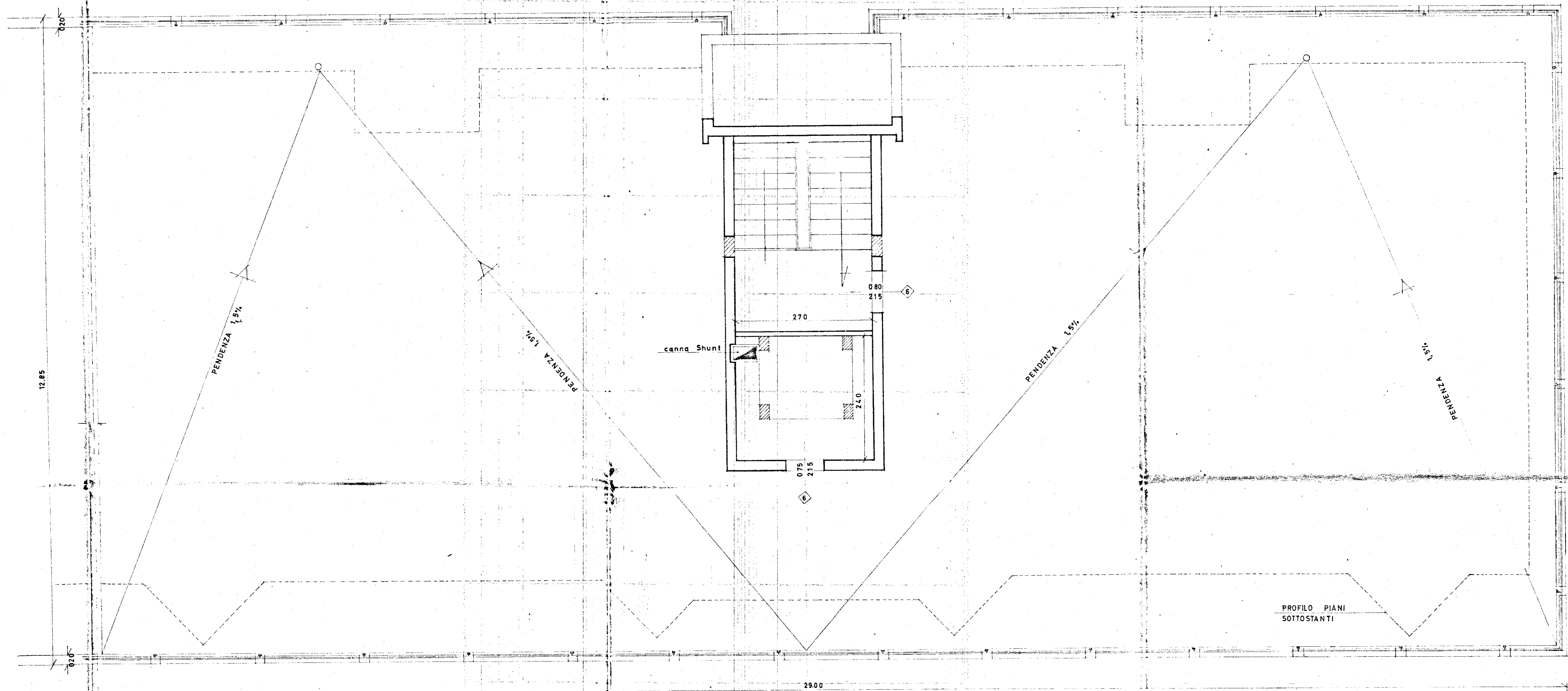
PIANTA TERRAZZE
