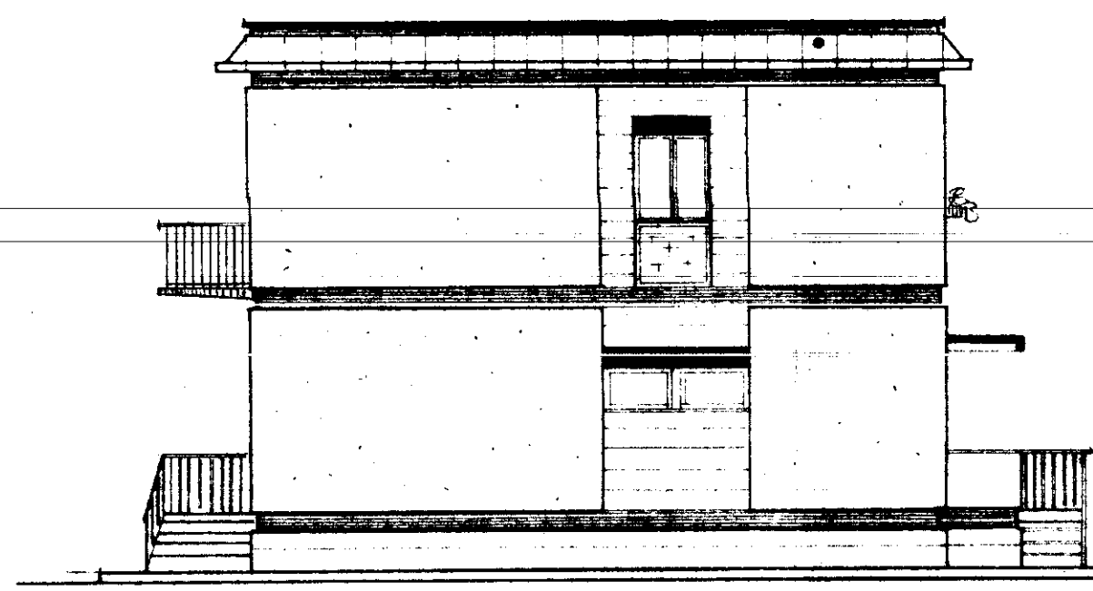
TESTATA A-D
