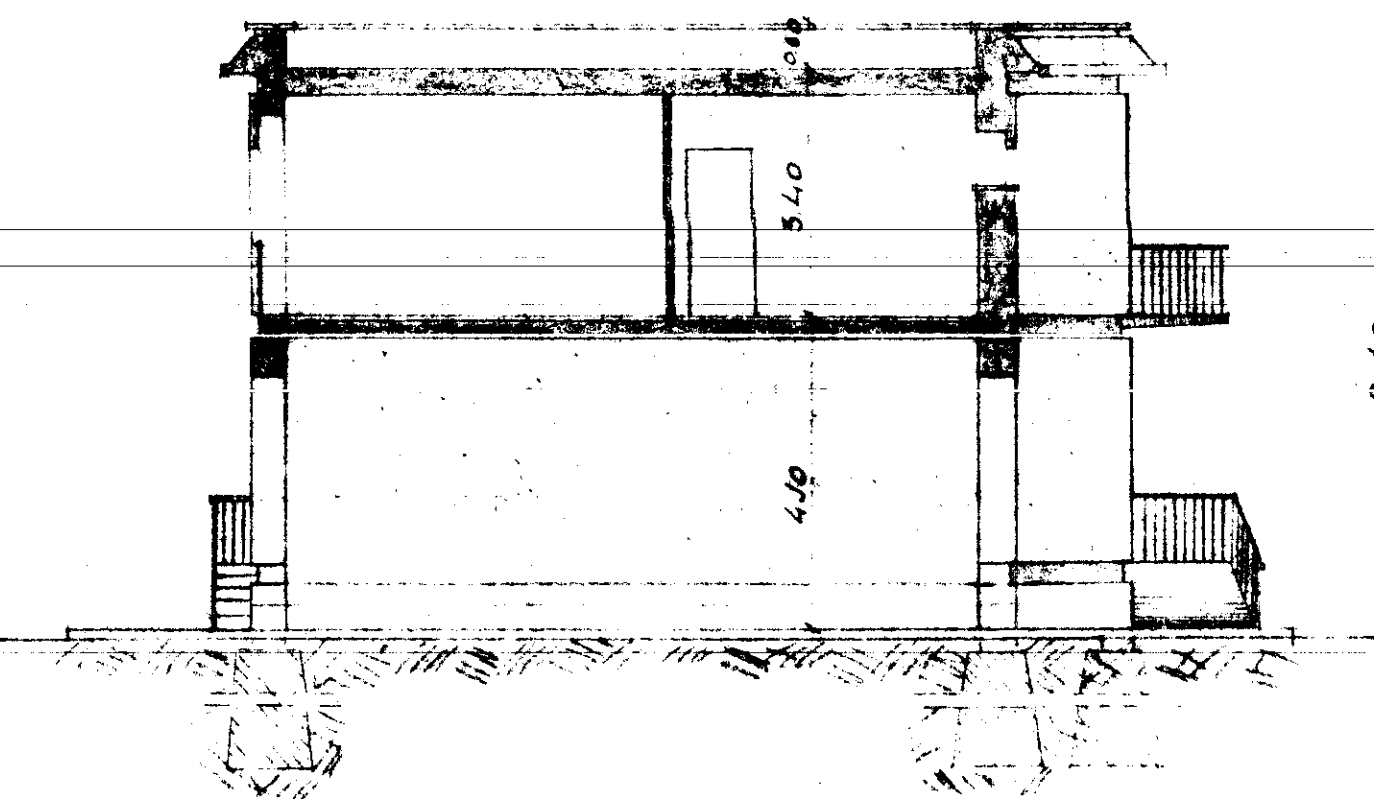
SEZIONE F-F'
