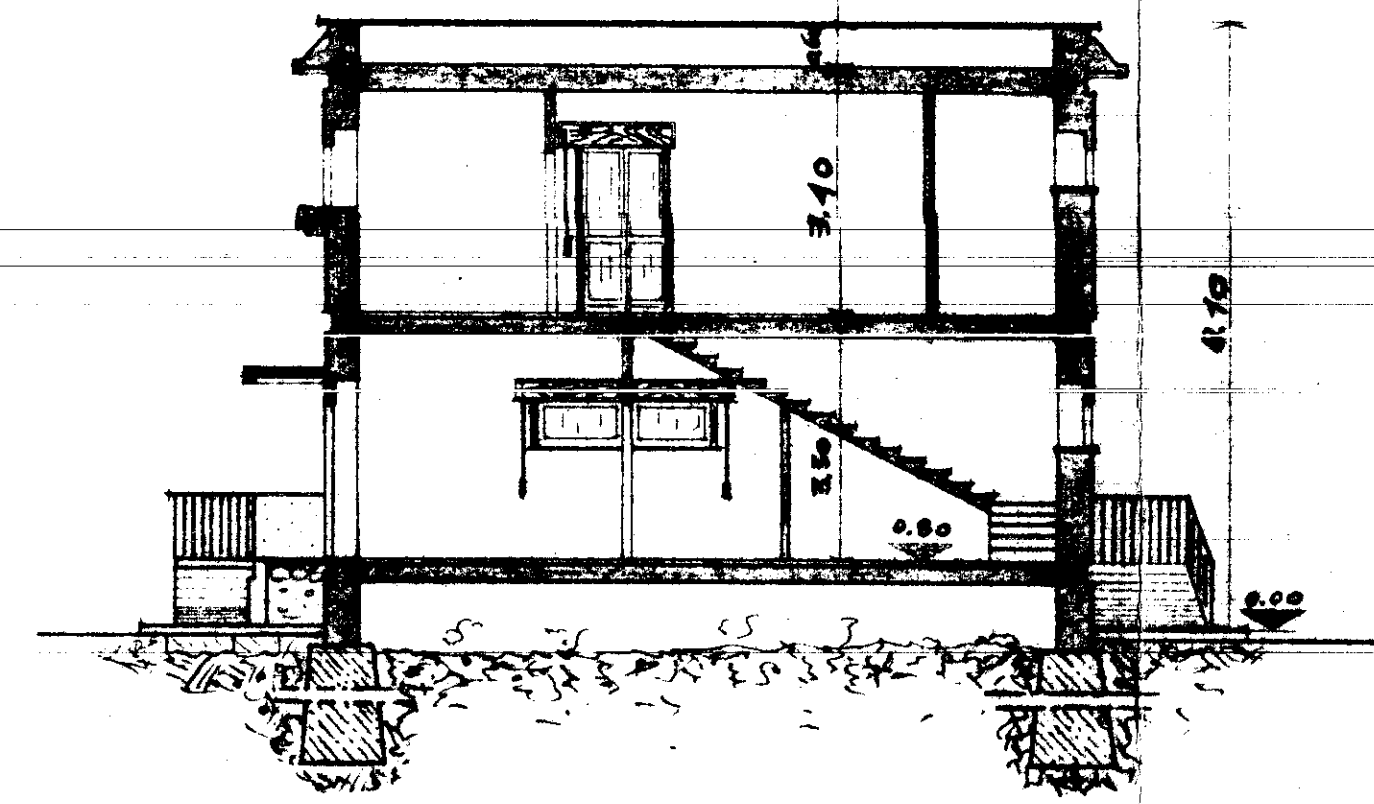
SEZIONE E-E'
