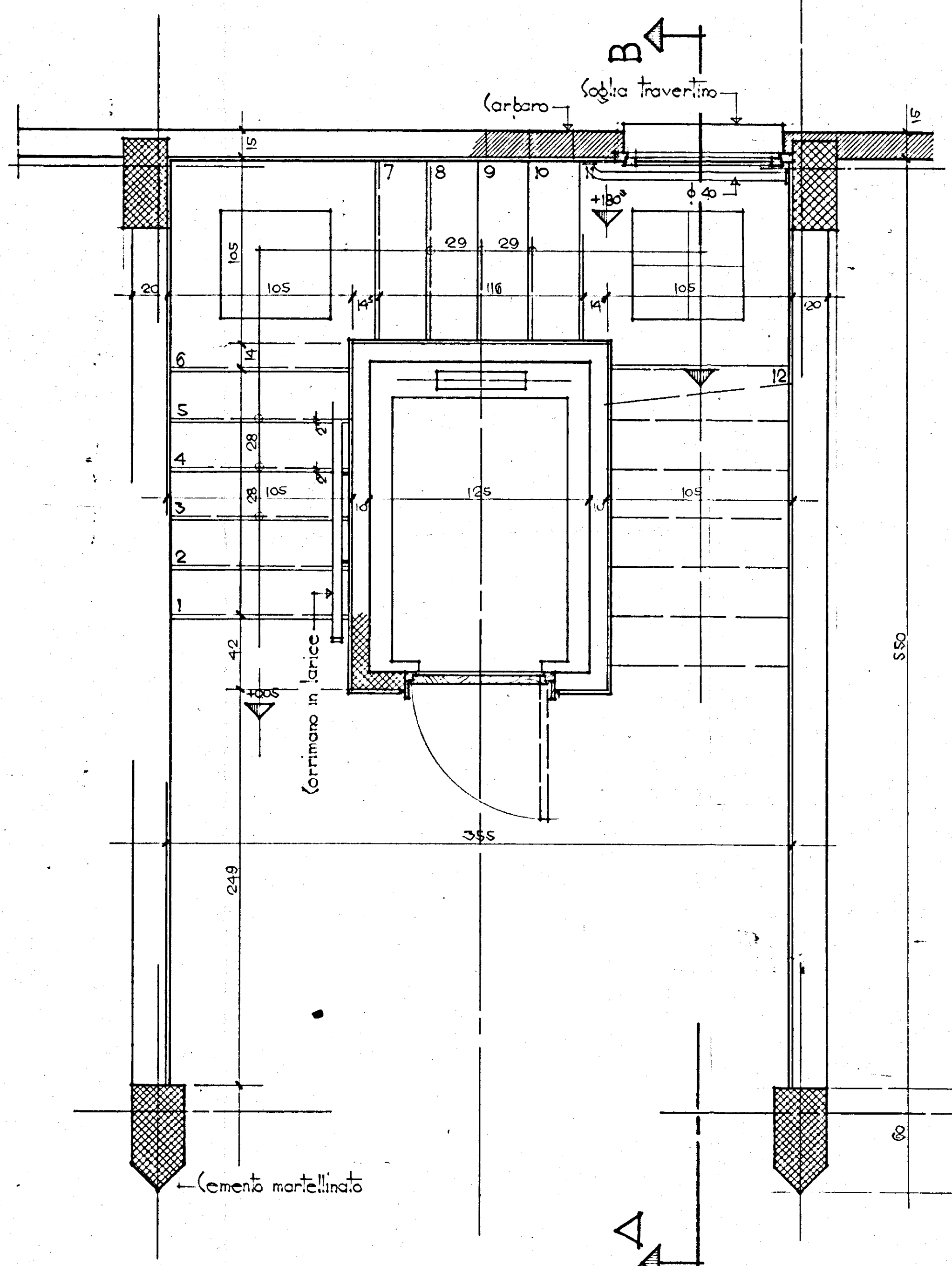
PIANTA PIANOTERRA
