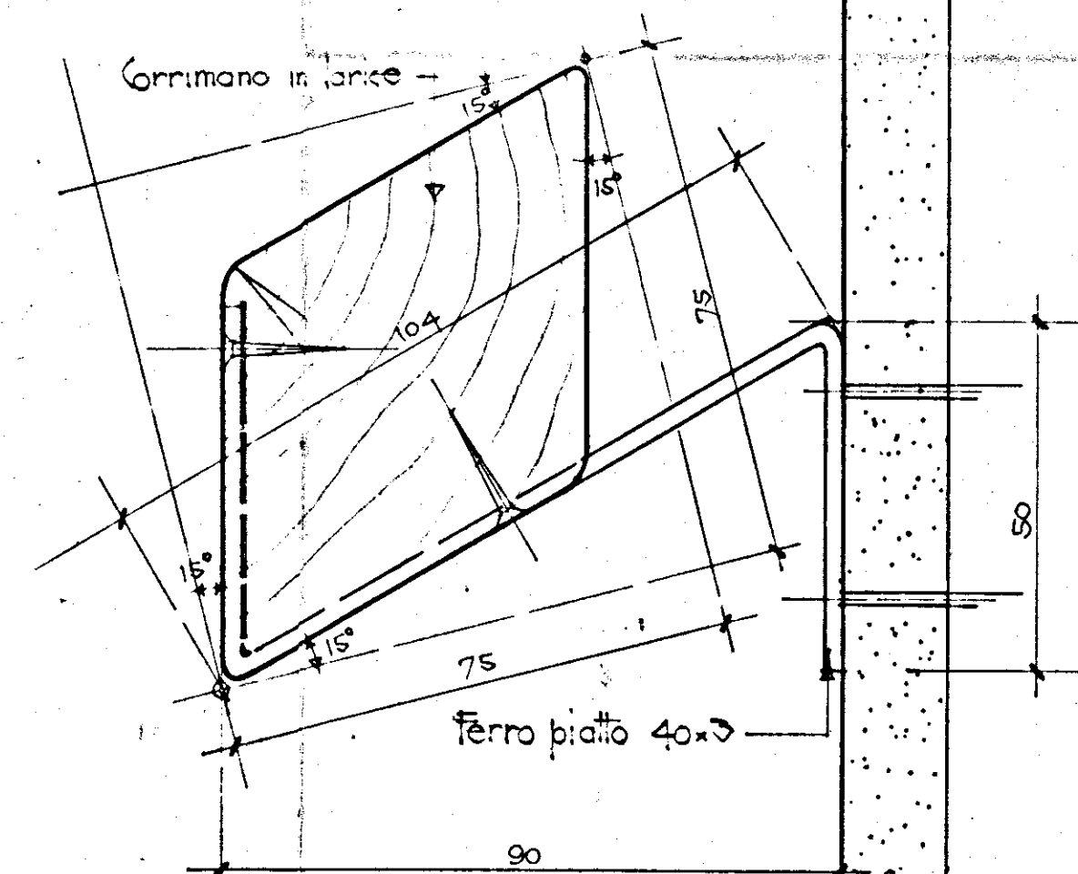
PARTICOLARE CORRIMANO rapp. 1:1
