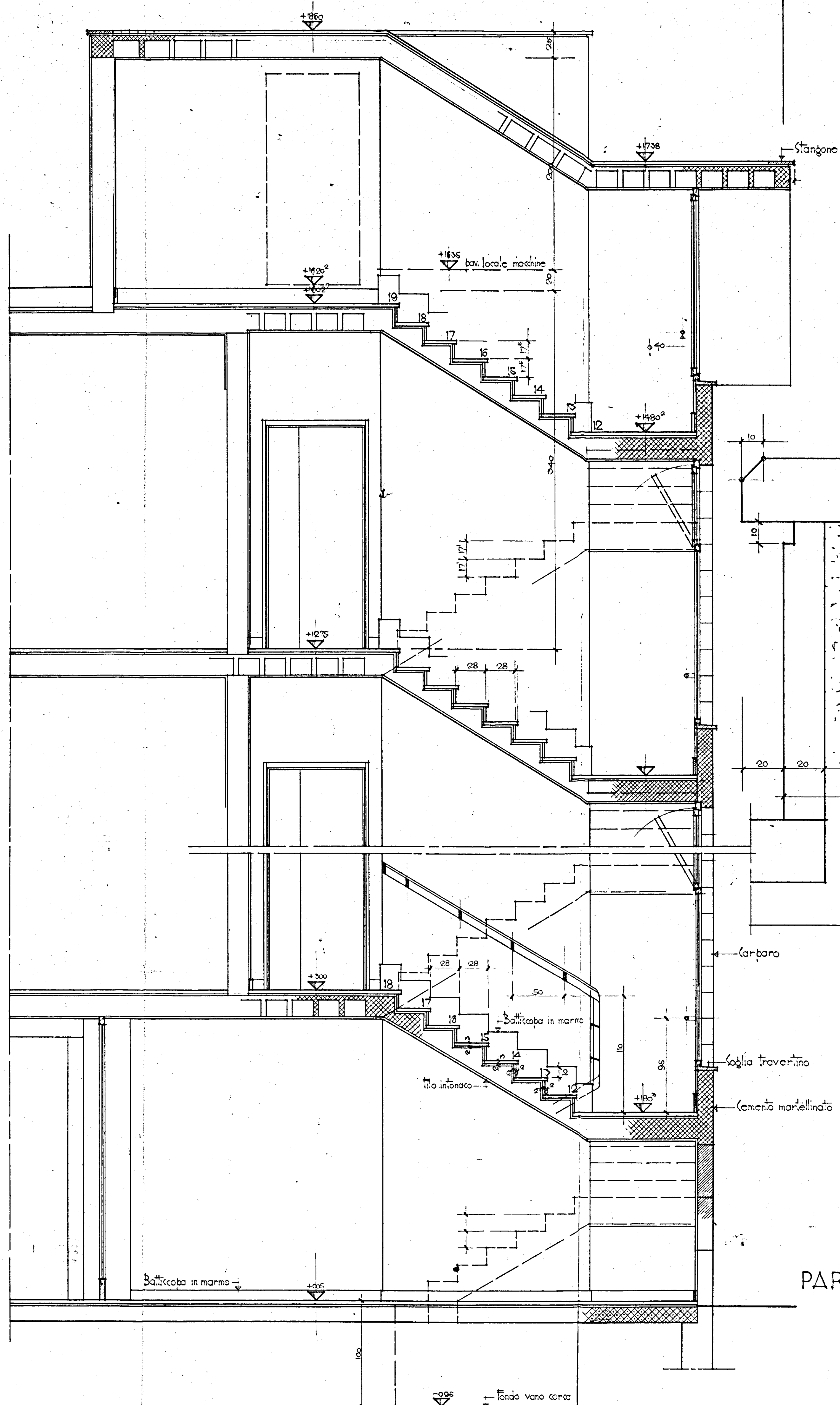
SEZIONE A-B
