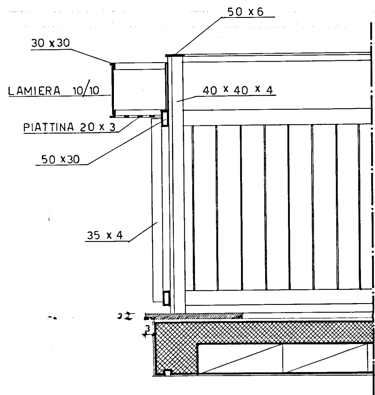
SEZIONE A-B RAPP. 1:10
