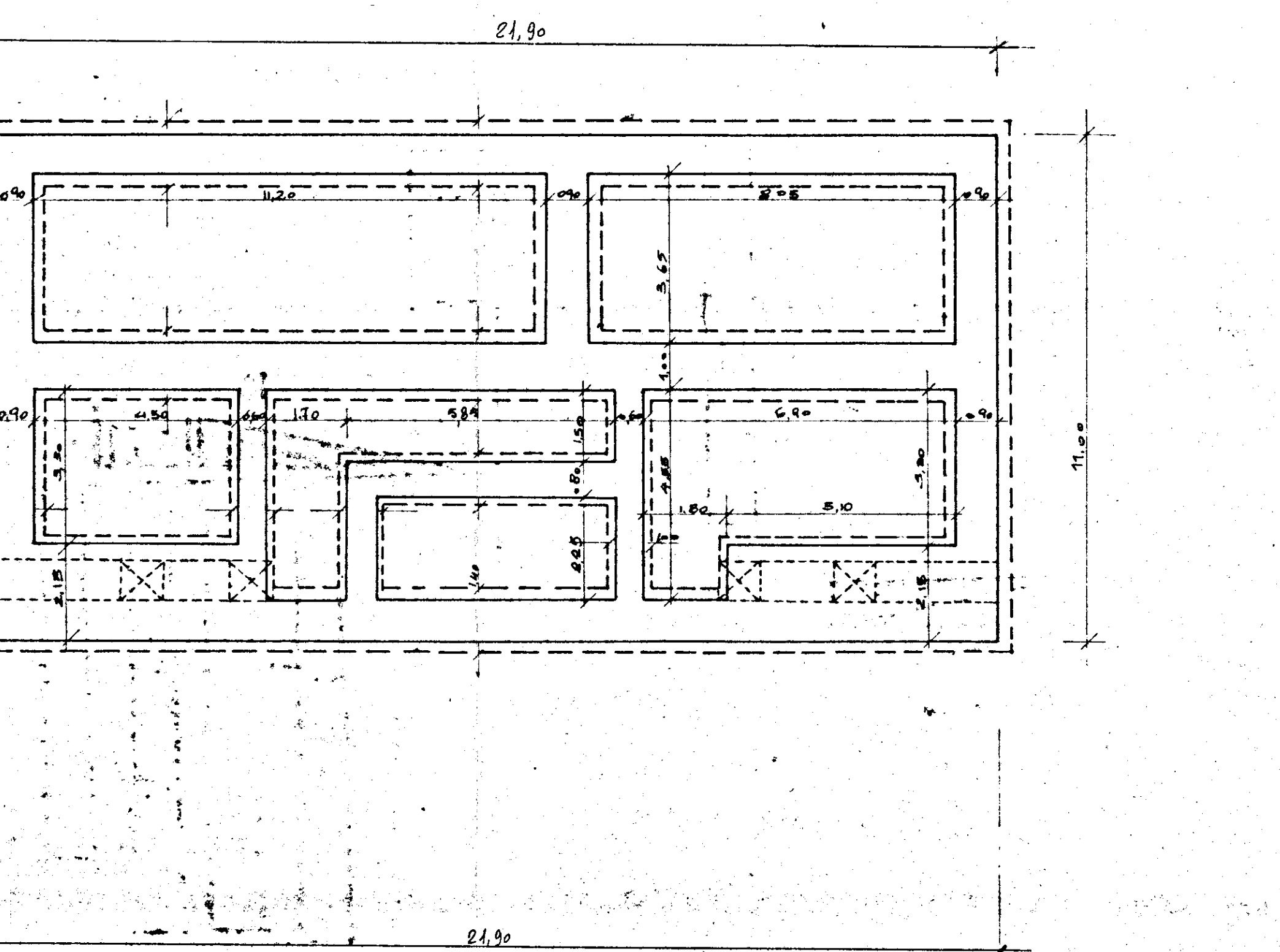
PIANTA FONDAZIONI
