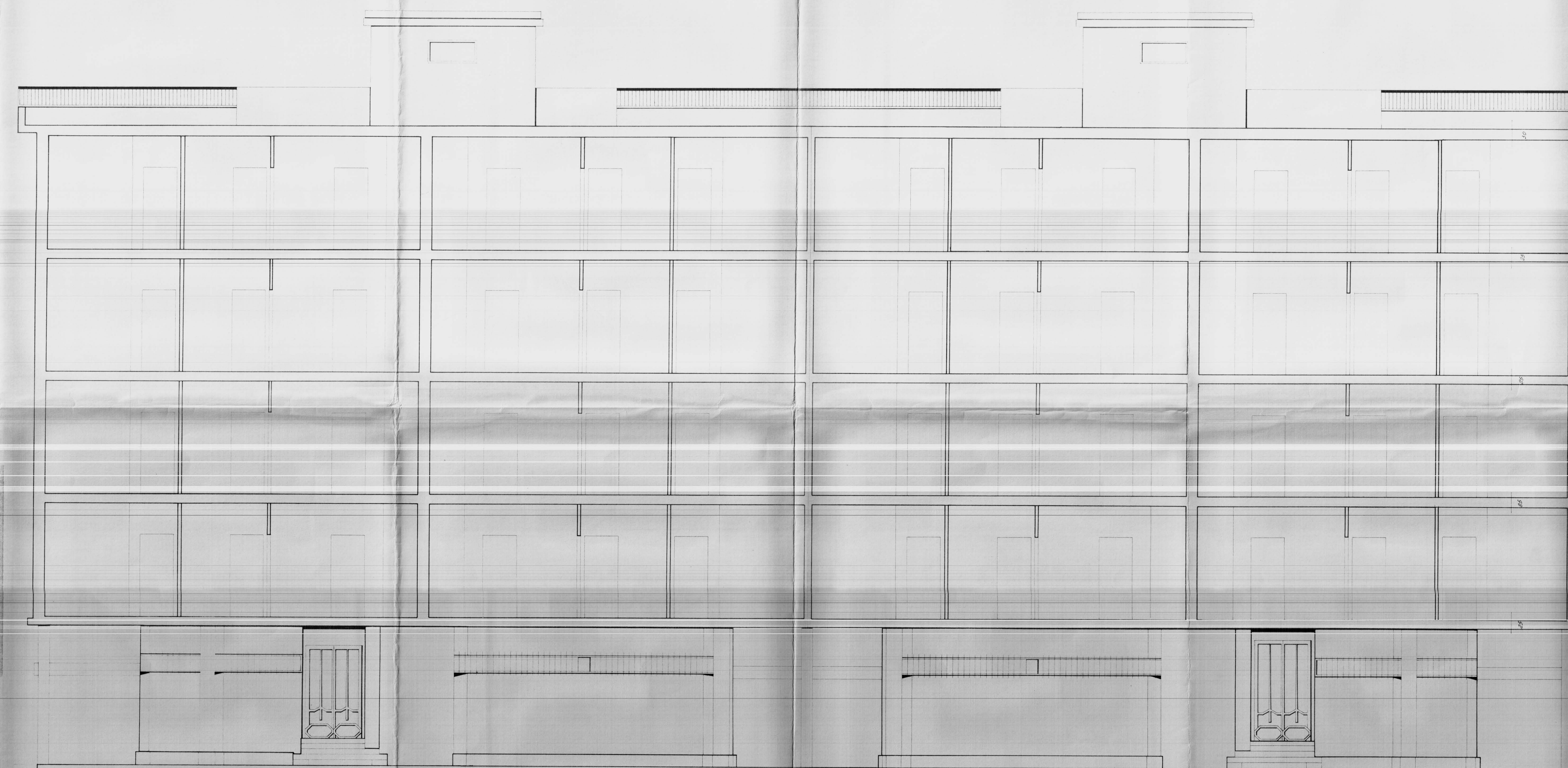
- SEZIONE A-B -
