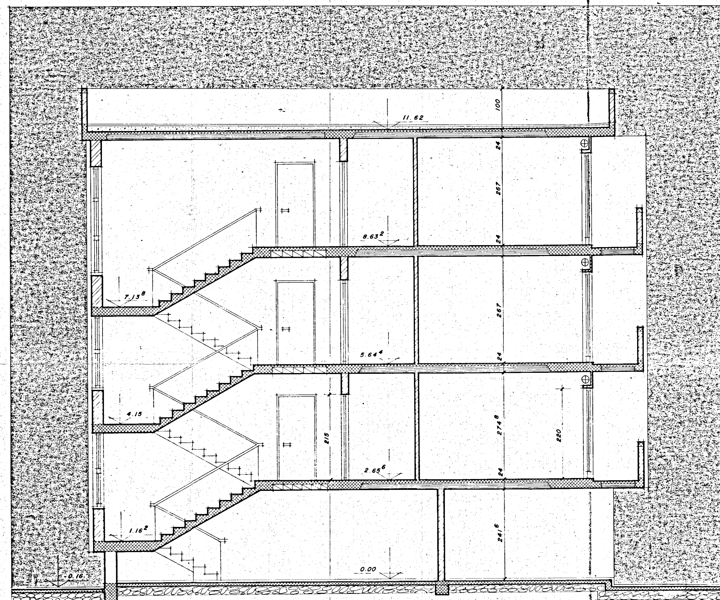
SEZIONE X-X
