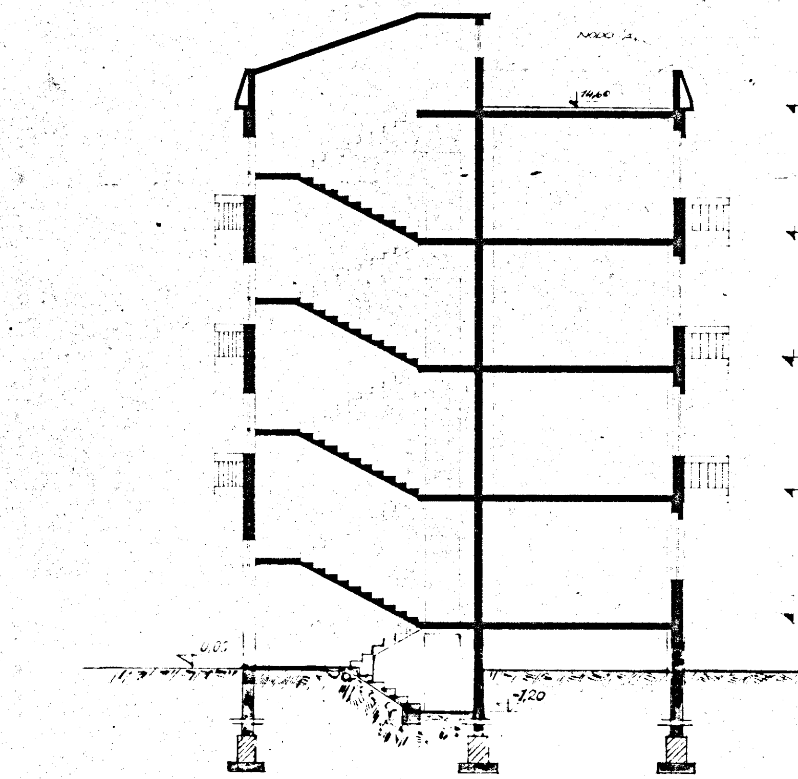
SEZIONE X-X
