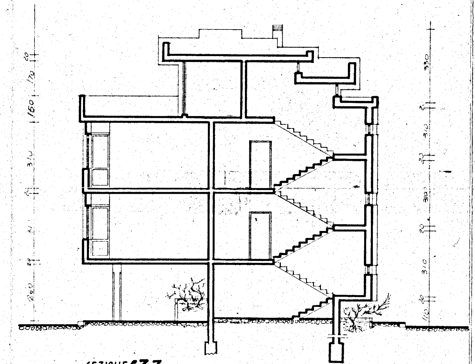
SEZIONE "ZZ"
