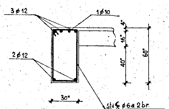
Sezione D-D
