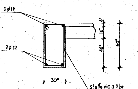
Sezione E-E
