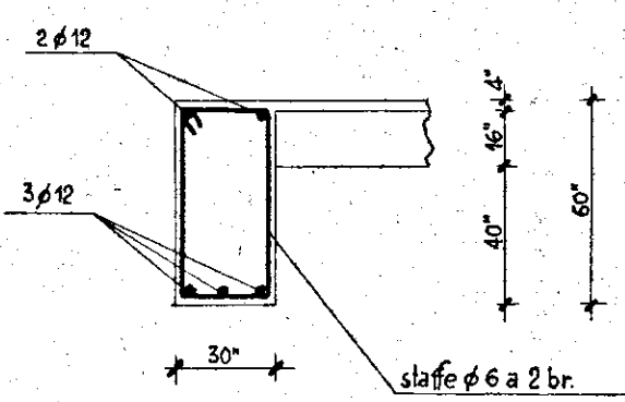
Sezione C-C
