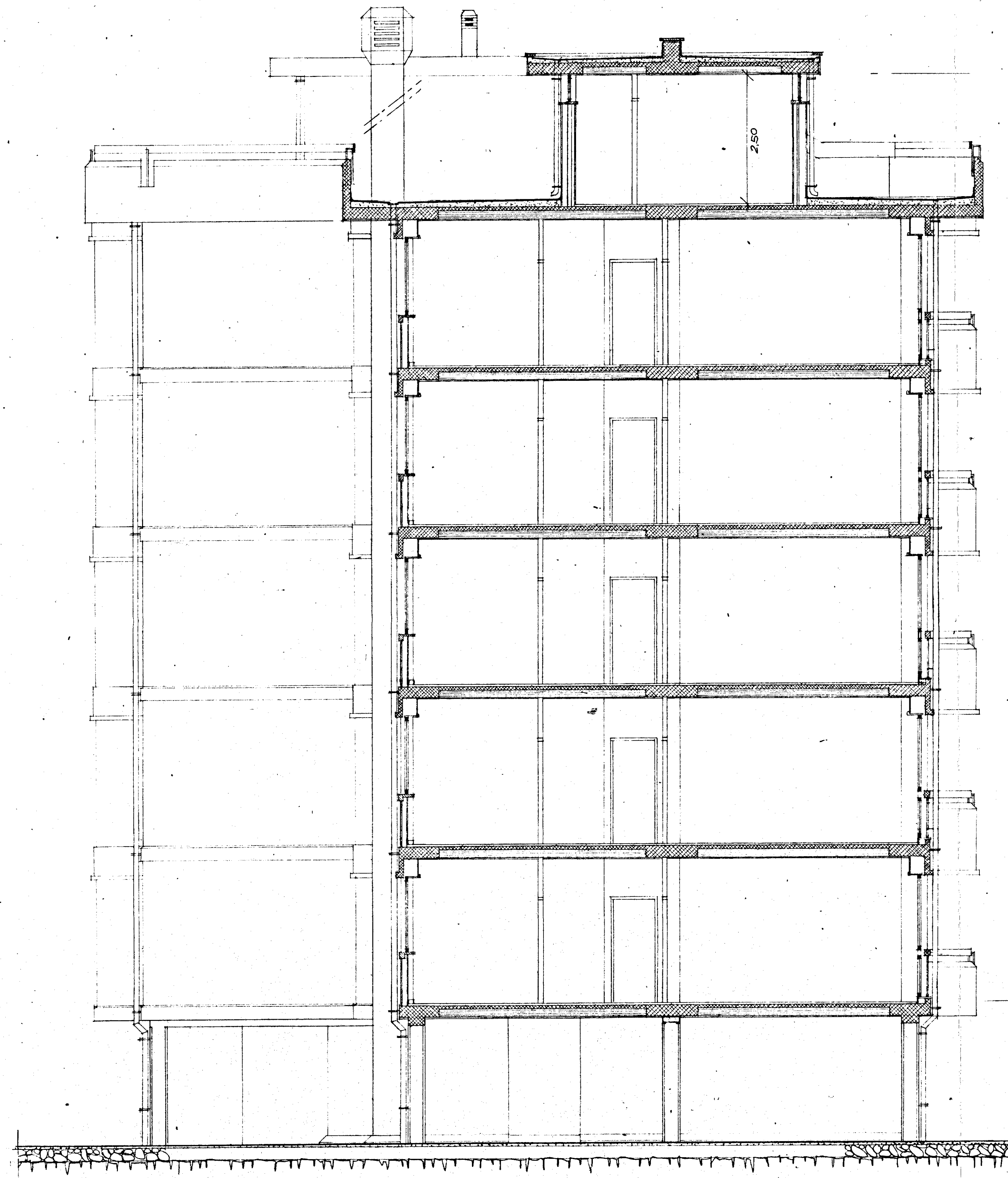
SEZIONE X-X
