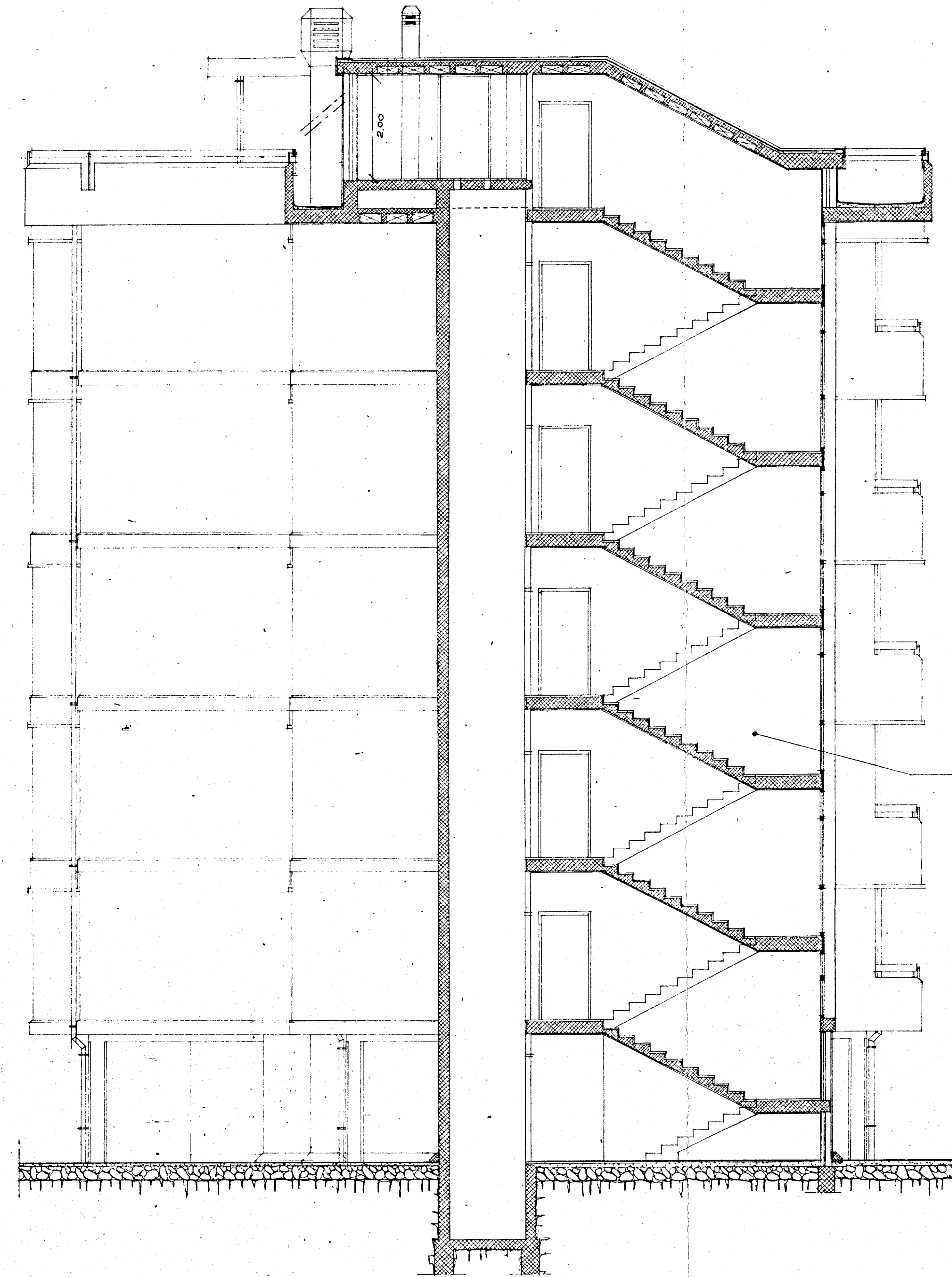
SEZIONE Y-Y
