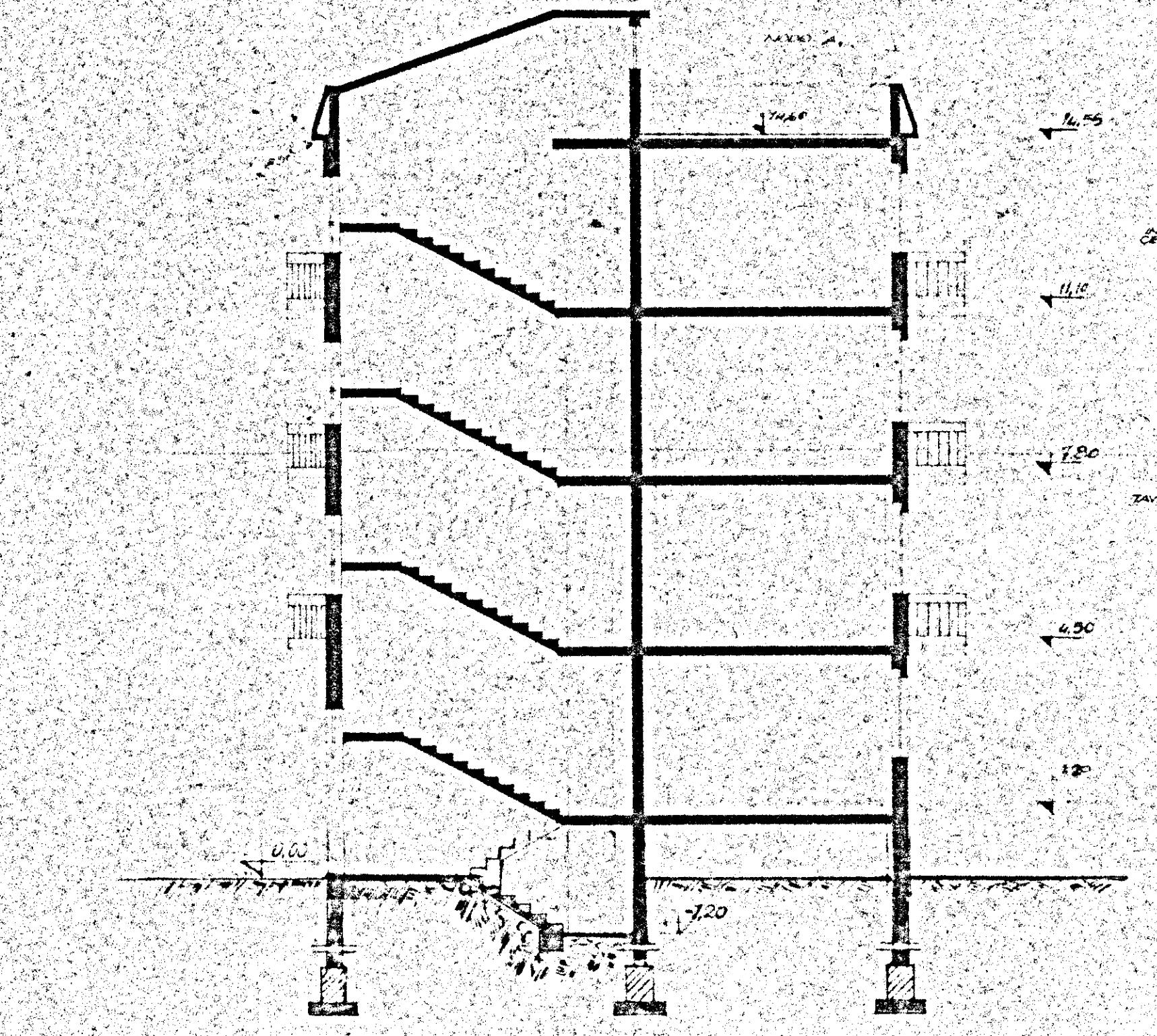
SEZIONE X-X
