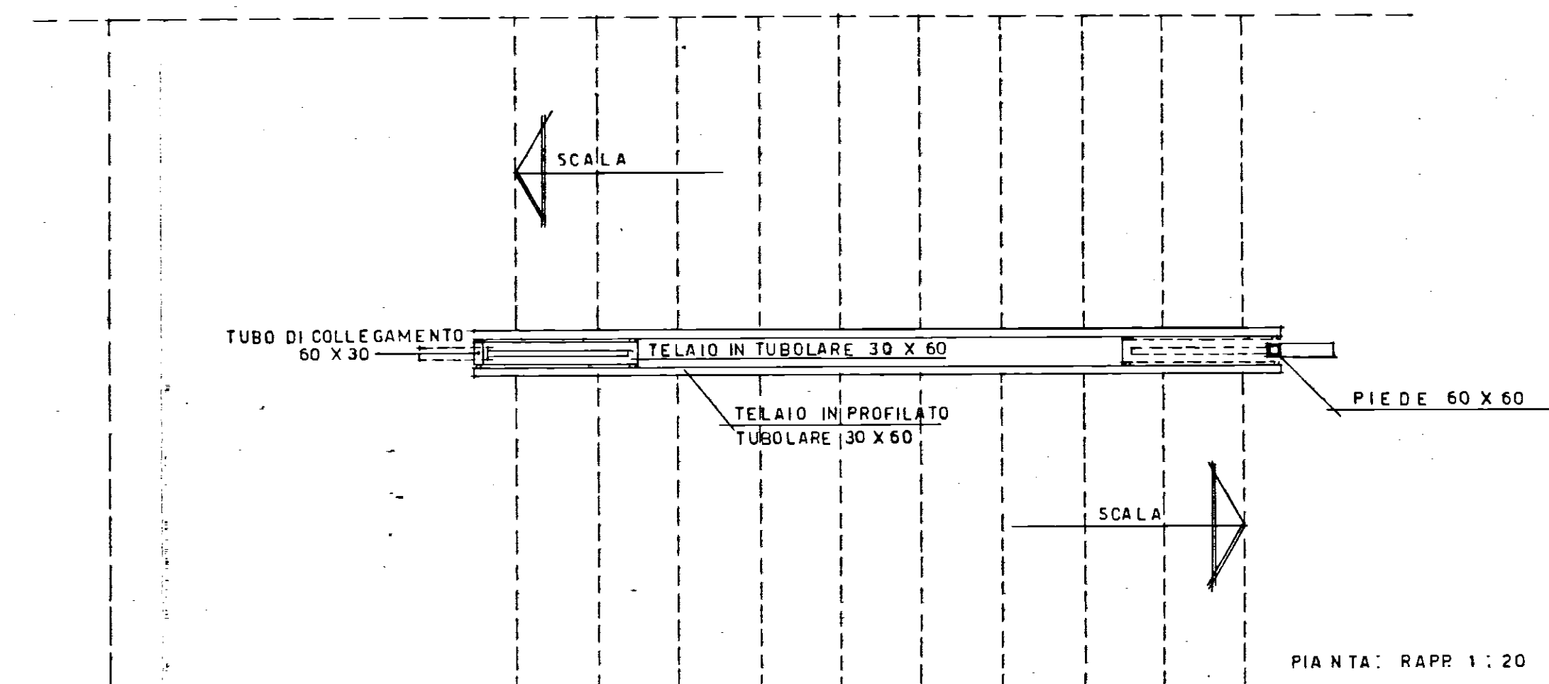
PARTICOLARI 1:20 RINGHIERA SCALA
