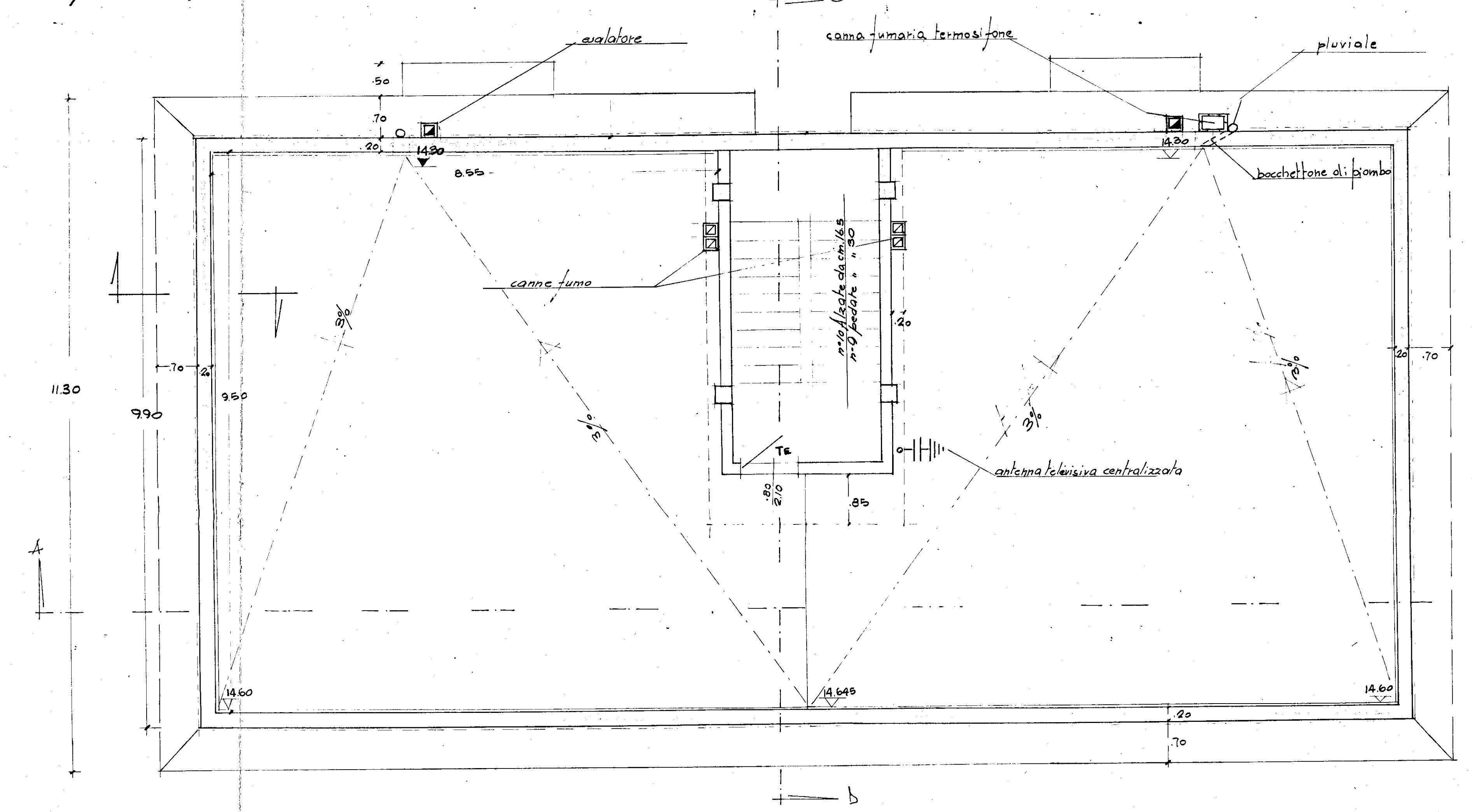
pianta coperture
