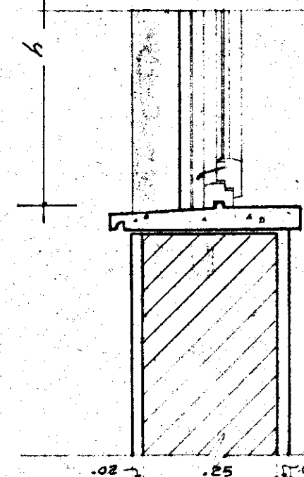
SEZIONE TIPO VETRA
