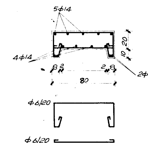
SEZIONE TRAVE DI CORONAMENTO PORTICO RAPPO 1:20
