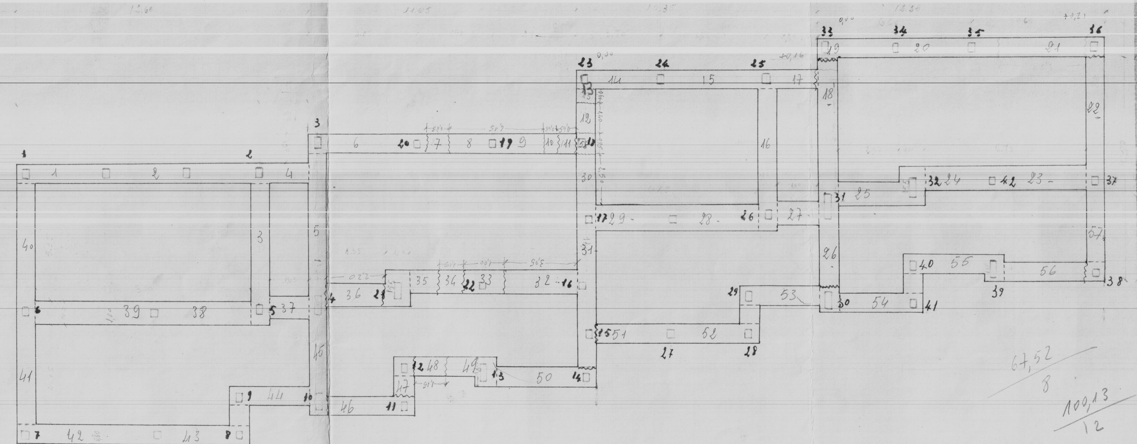
Pianta fondazione scala 1:100
