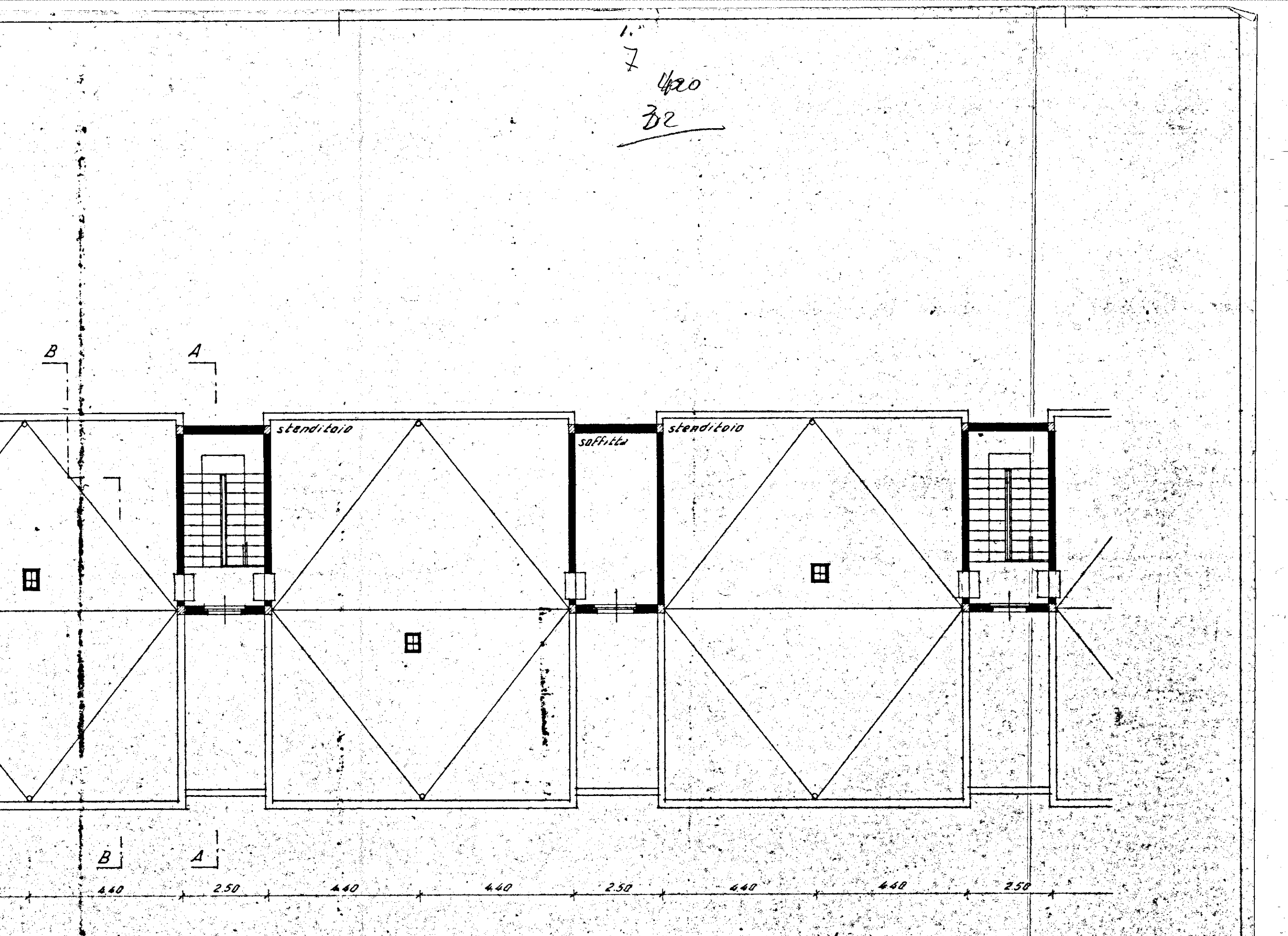
PIANTA DEL PIANO DELLE TERRAZZE DI COPERTURA
