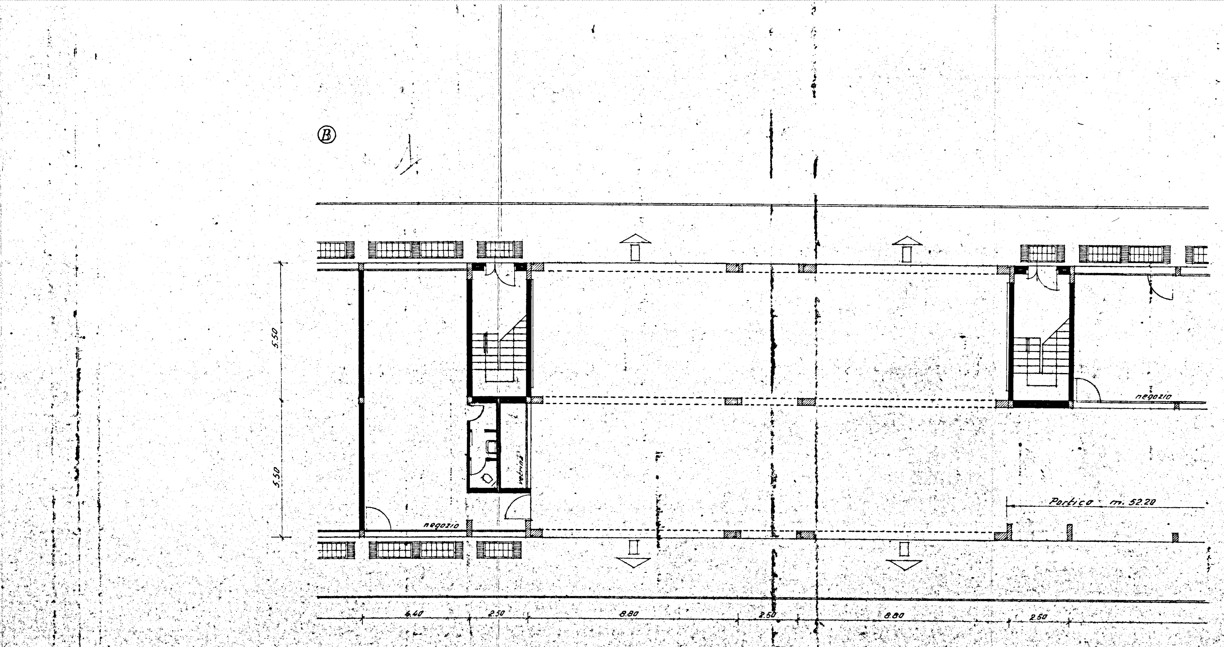
PIANTA DEL PIANO TERRENO IN CORRISPONDENZA DEL PASSAGGIO PEDONALE E INIZIO PORTICO
