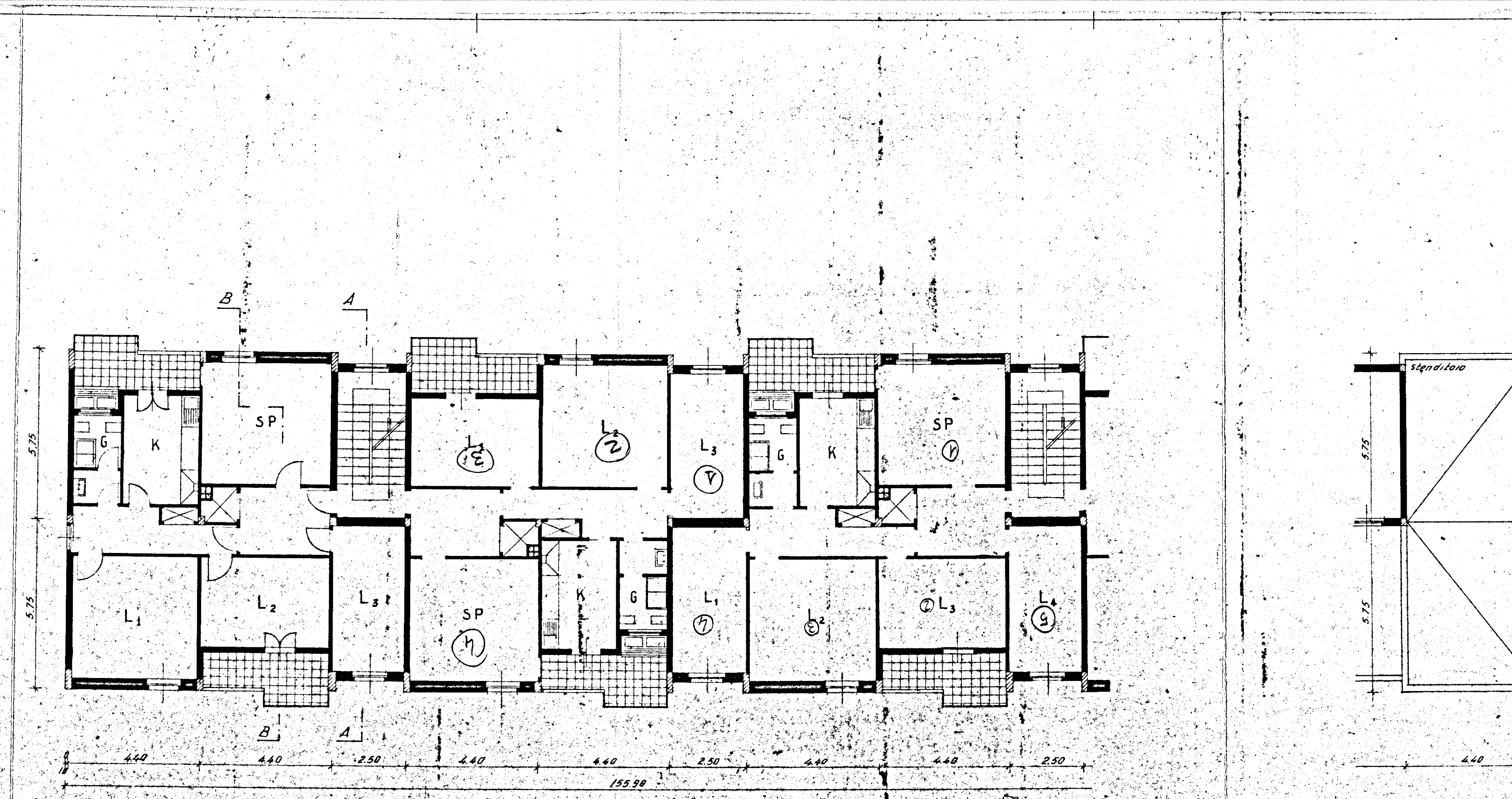
PIANTA DEL PIANO TIPO
