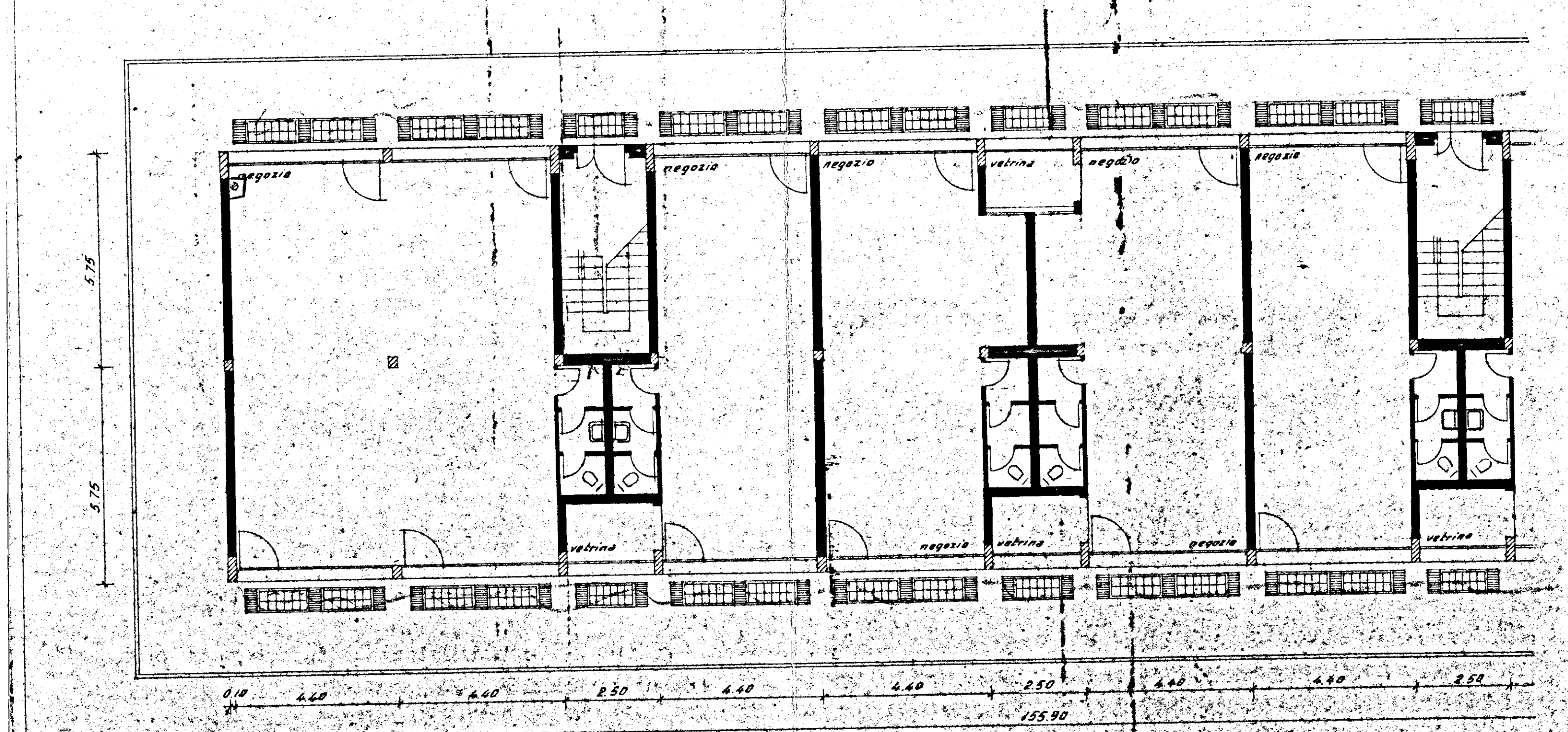
PIANTA DEL PIANO TERRENO
