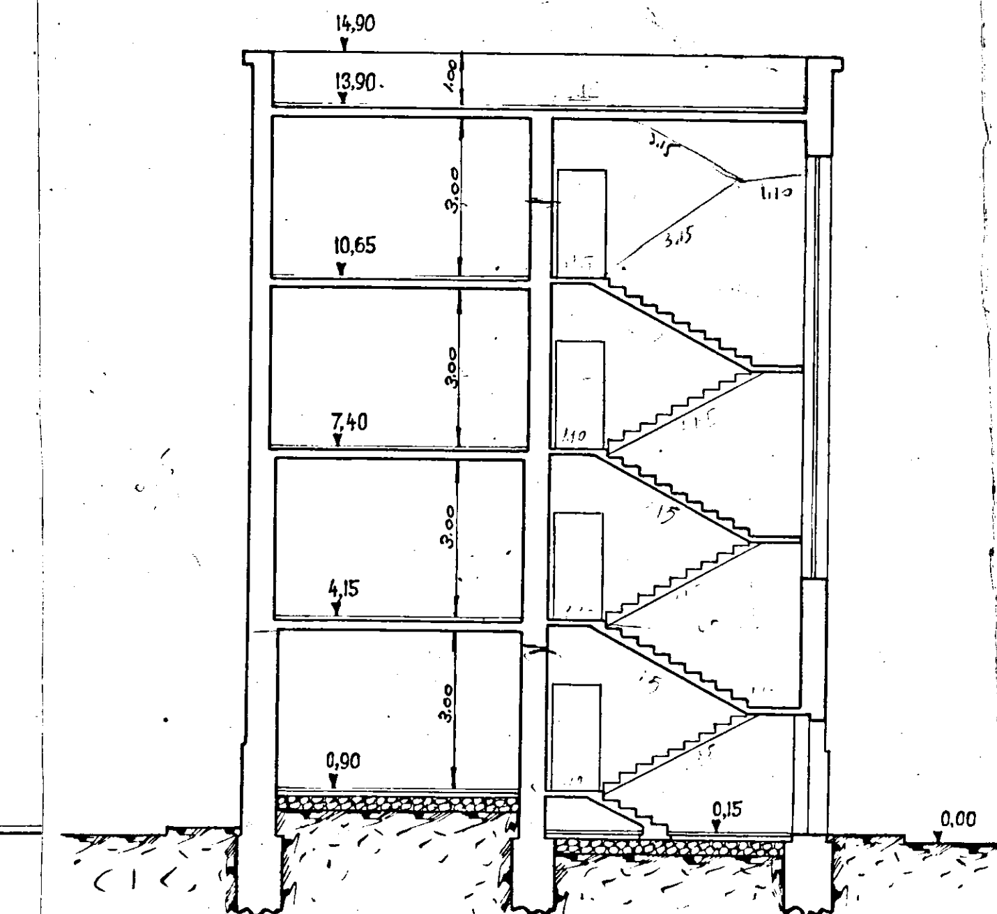
Sezione A-D
