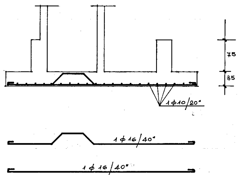
SEZIONE A-B
