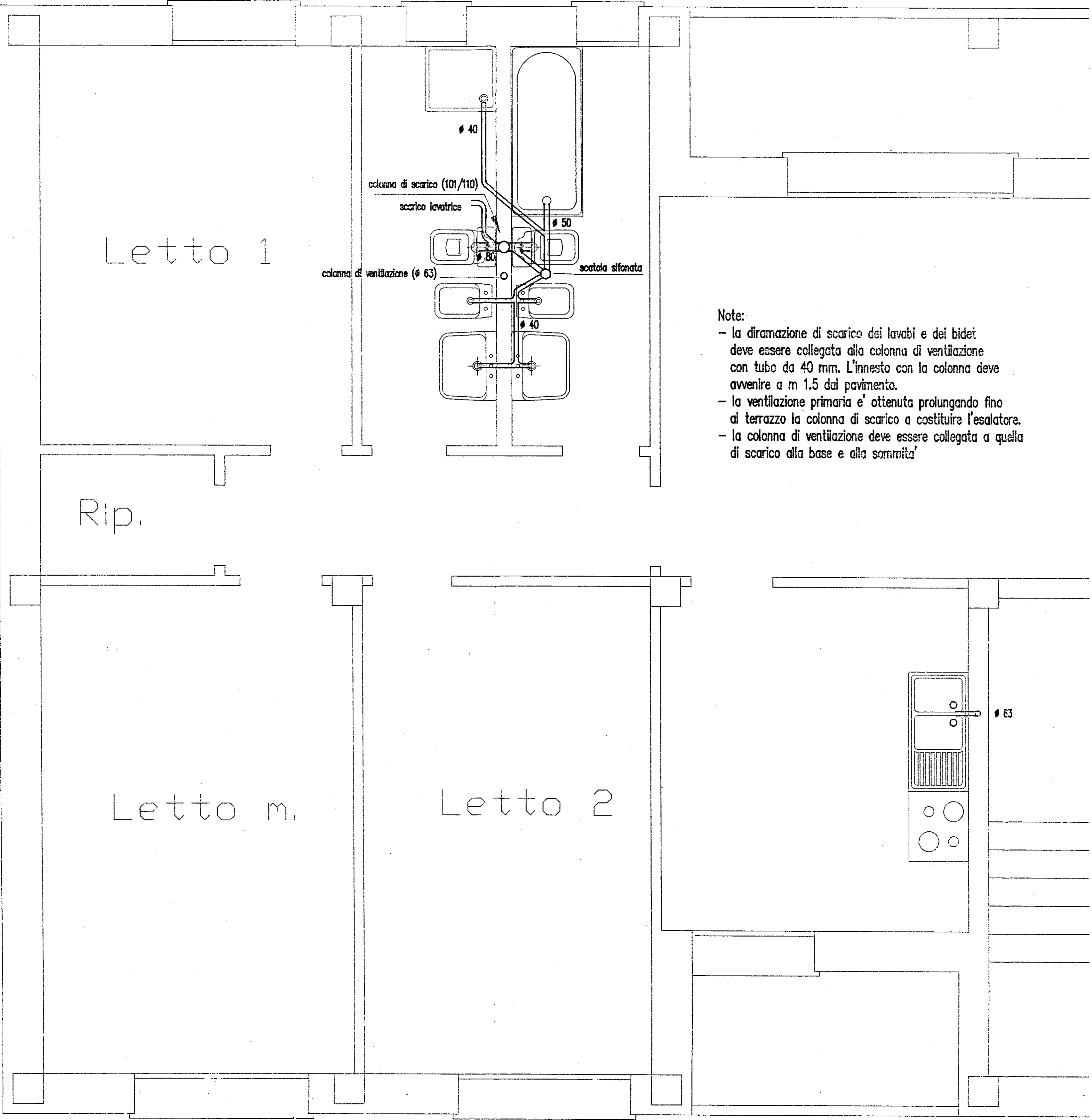
RETE DI SCARICO APPARTAMENTO TIPO – LOTTO 3 (Scala 1 : 25)
