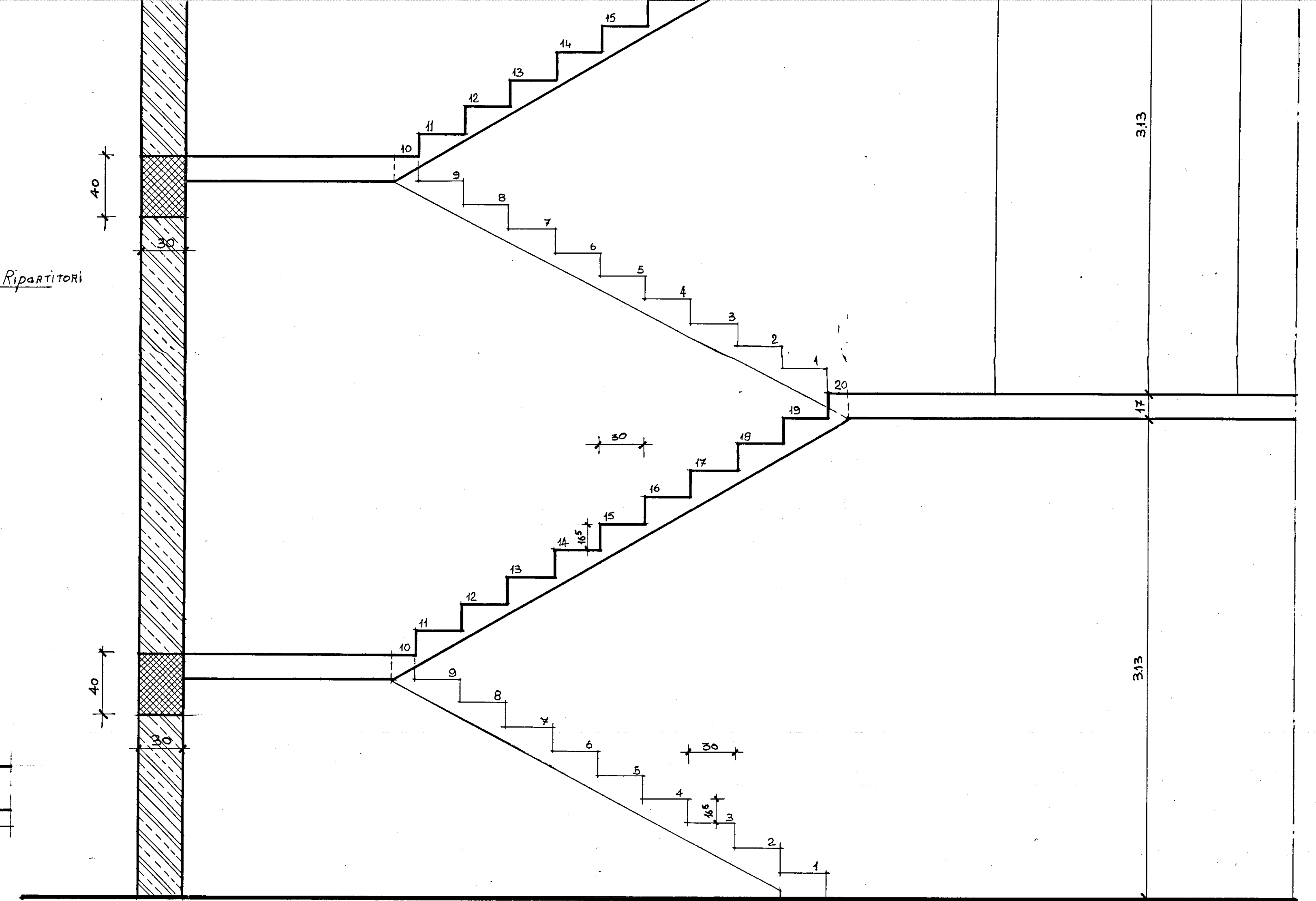
SEZIONE A-B
