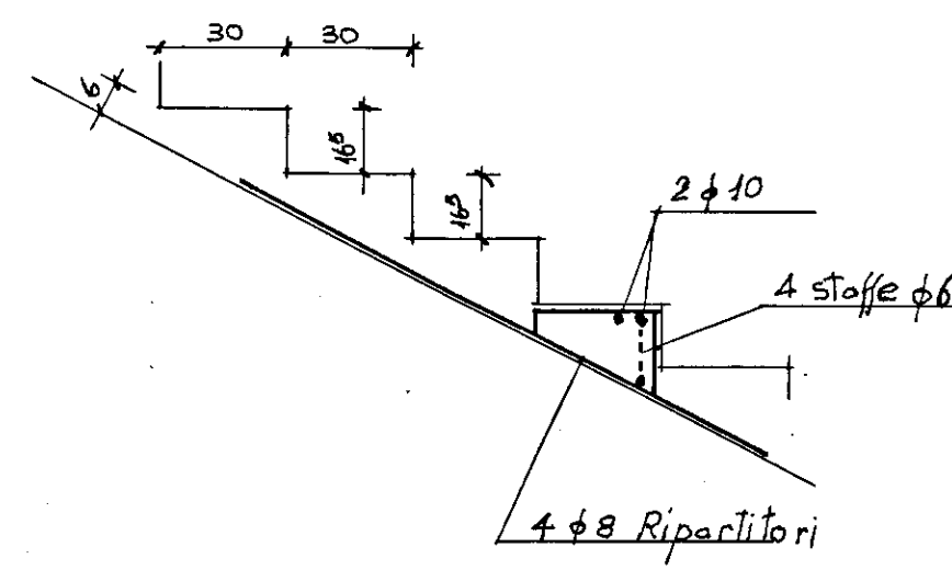
PARTICOLARE GRADINO
