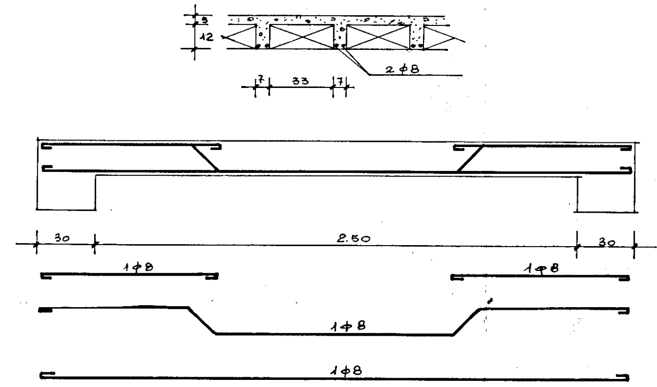
PARTICOLARE SOLAIO (A)
