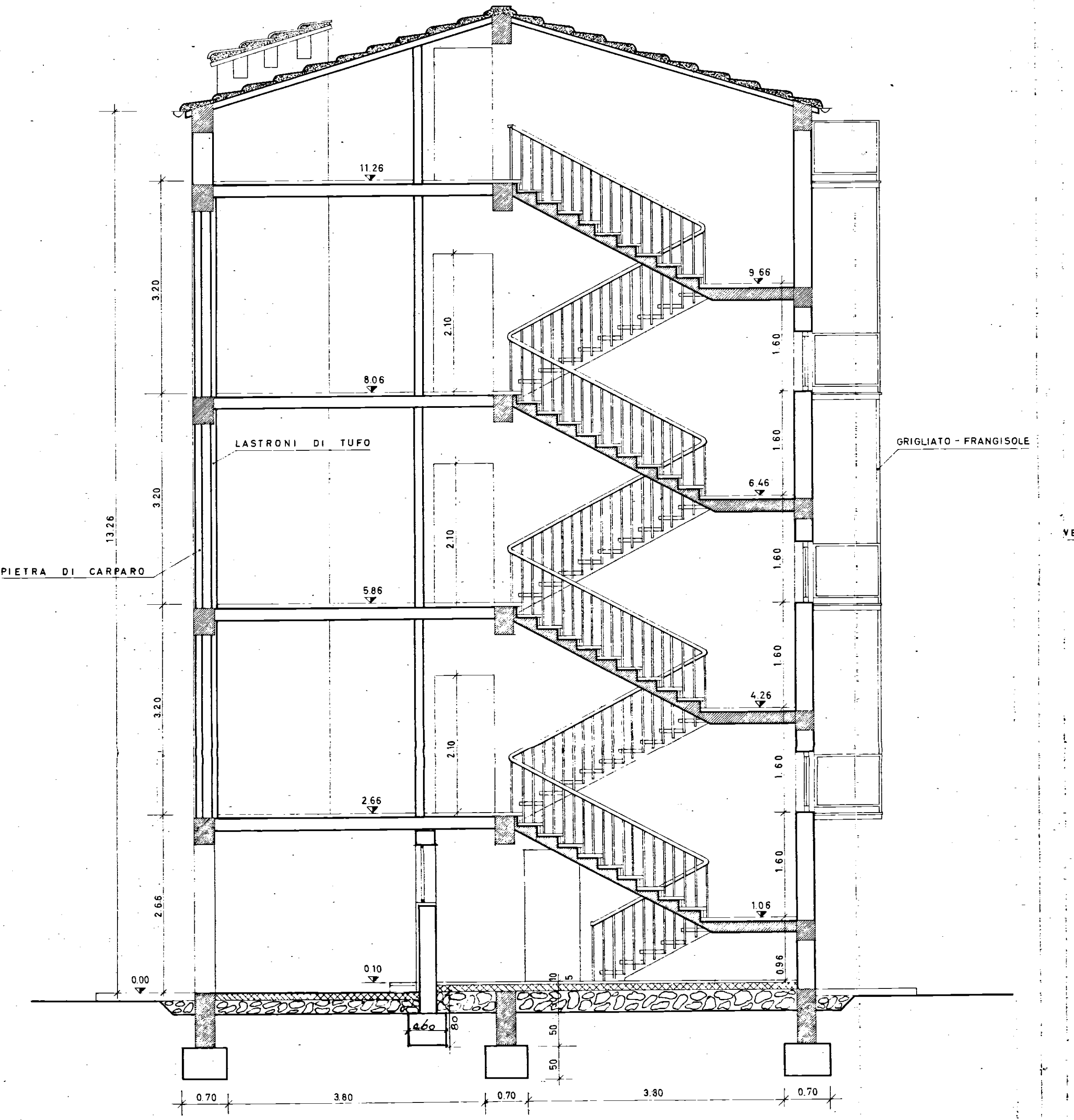
SEZIONE A - B
