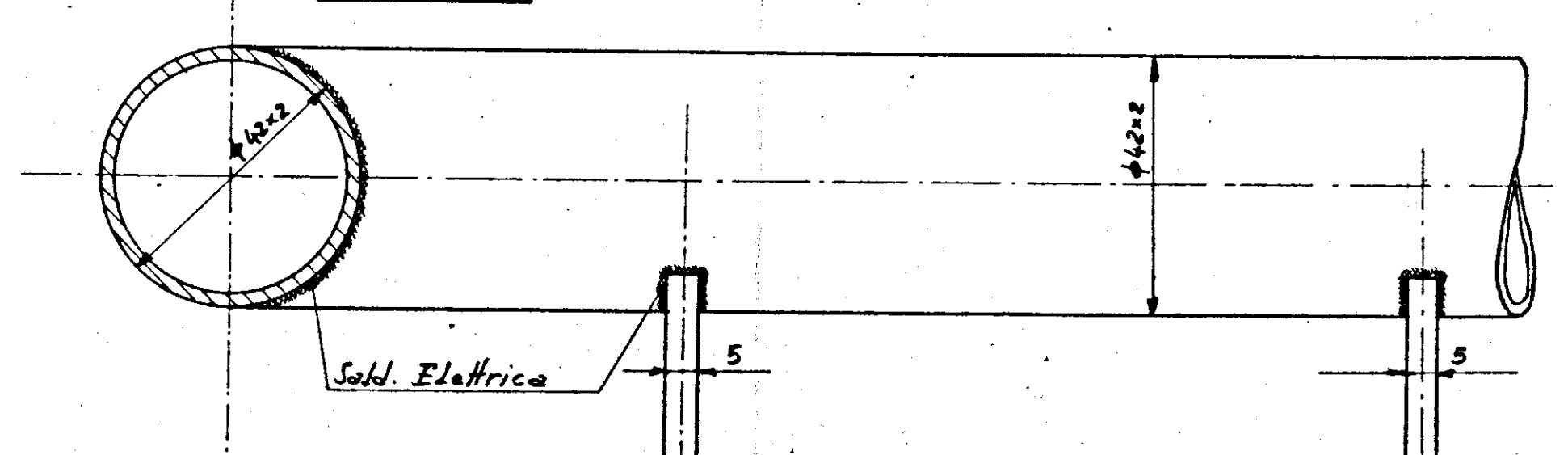
SEZ. AA SCALA 1:1
