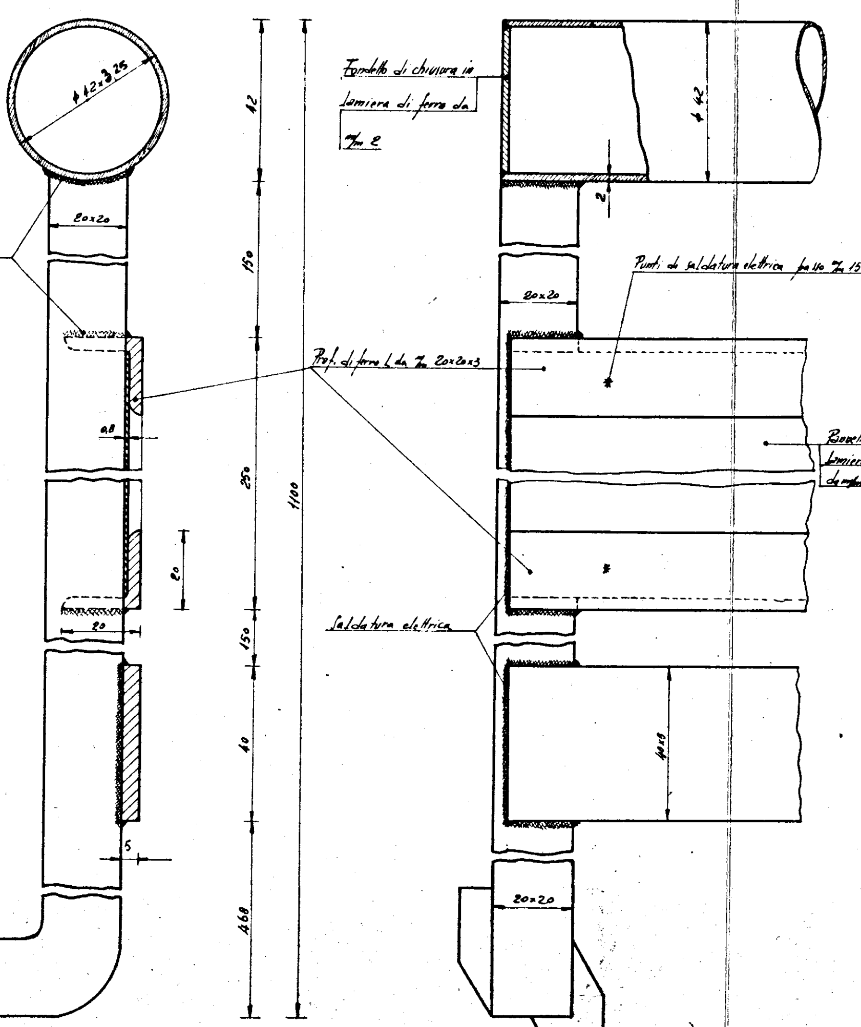
PARTICOLARE MONTANTE - SCALA 1:1
