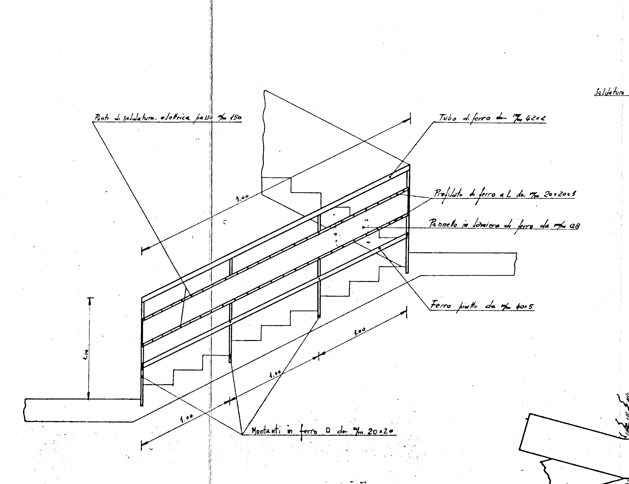
RINGHIERA PER SCALE SCALA 1:20
