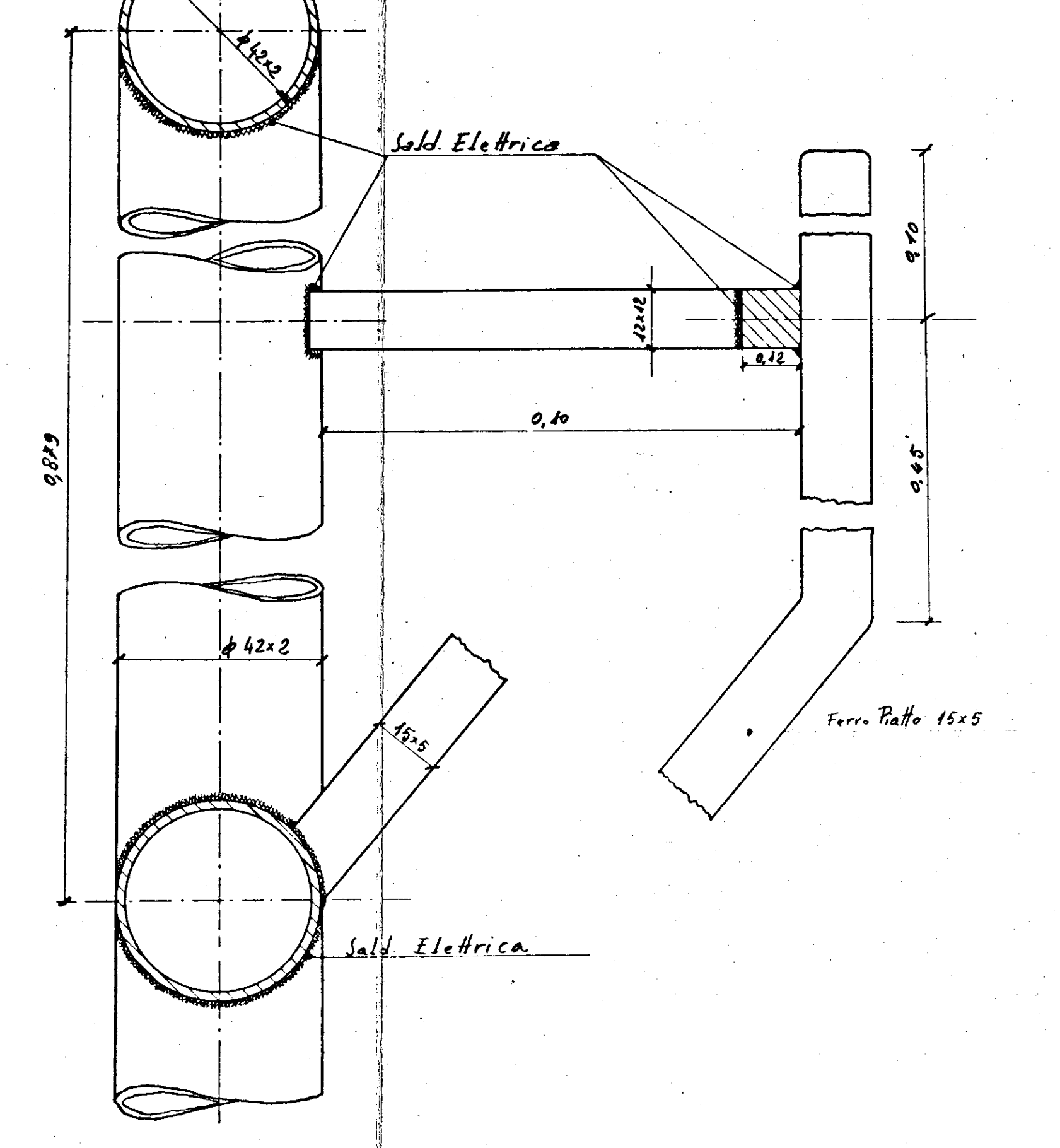
SEZ. BB SCALA 1:1
