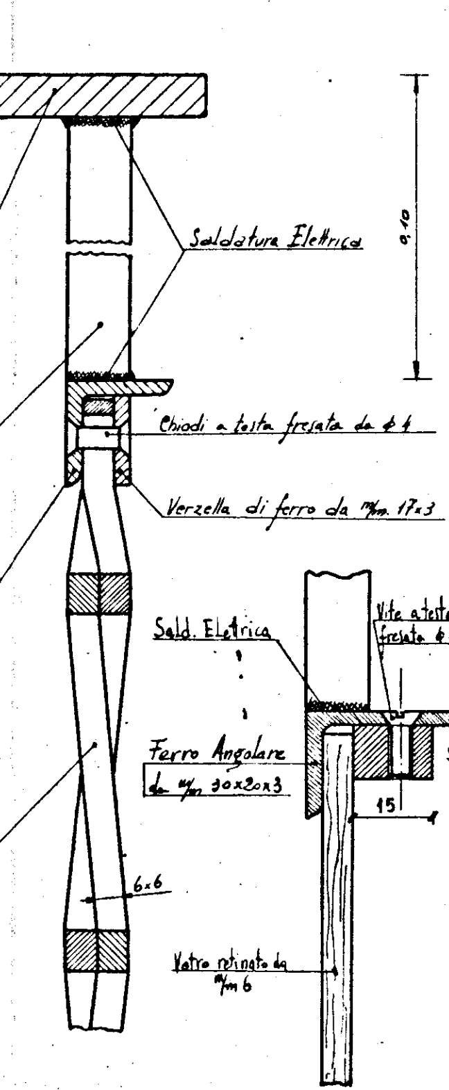
SEZ. AA SCALA 1:1
