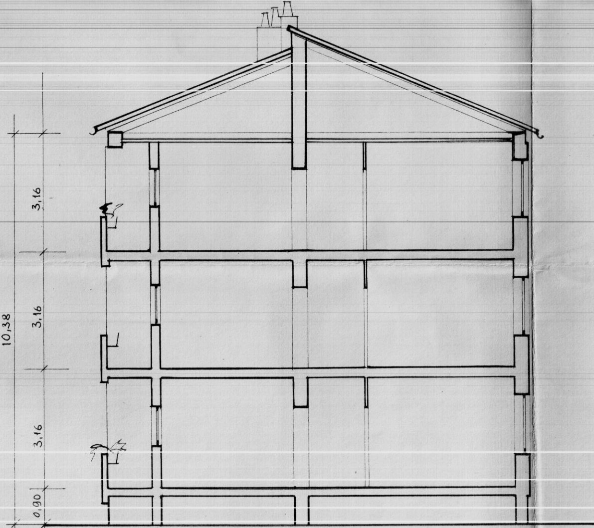
SEZIONE TRASVERSALE
