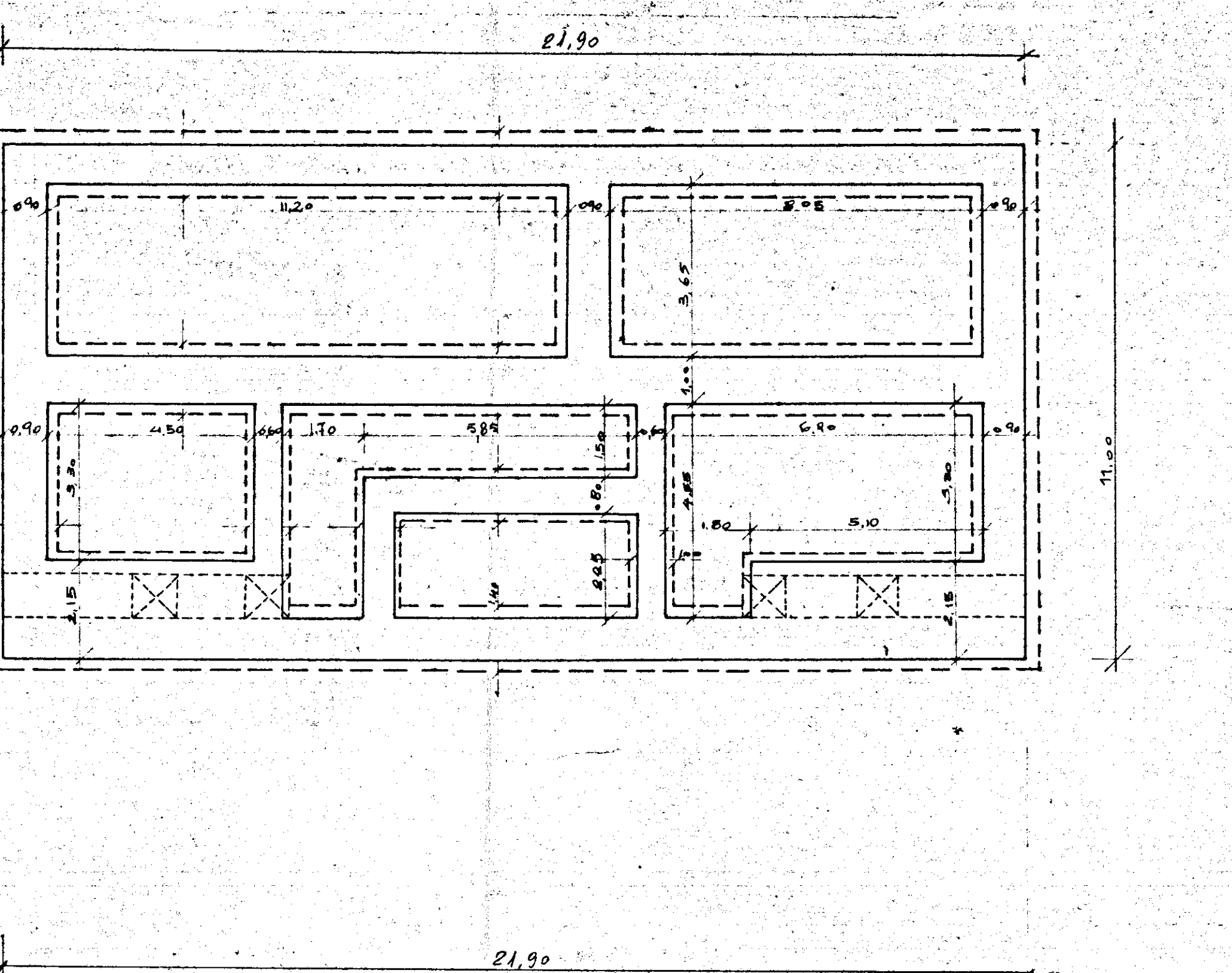
PIANTA FONDAZIONI
