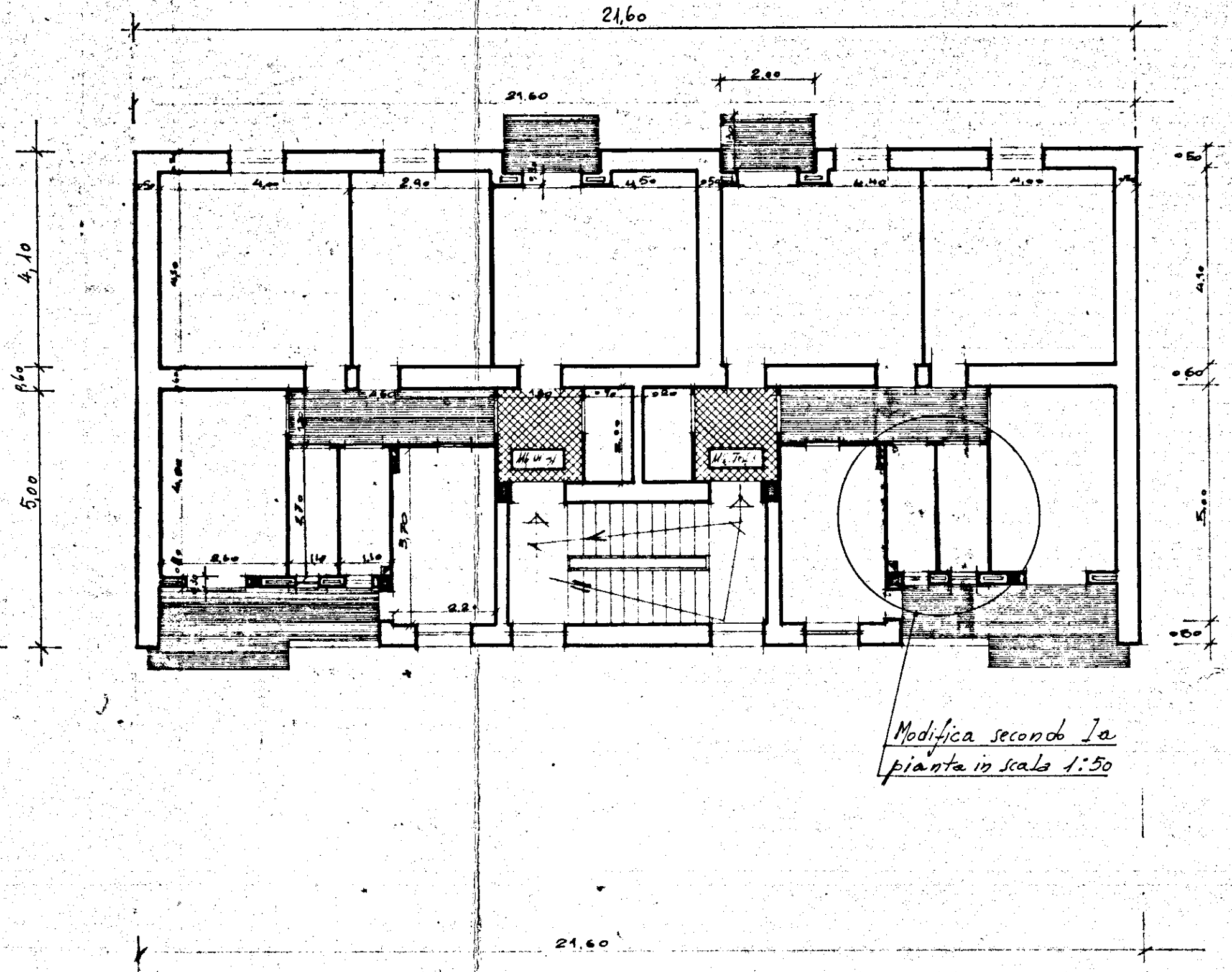
PRIMO PIANO
