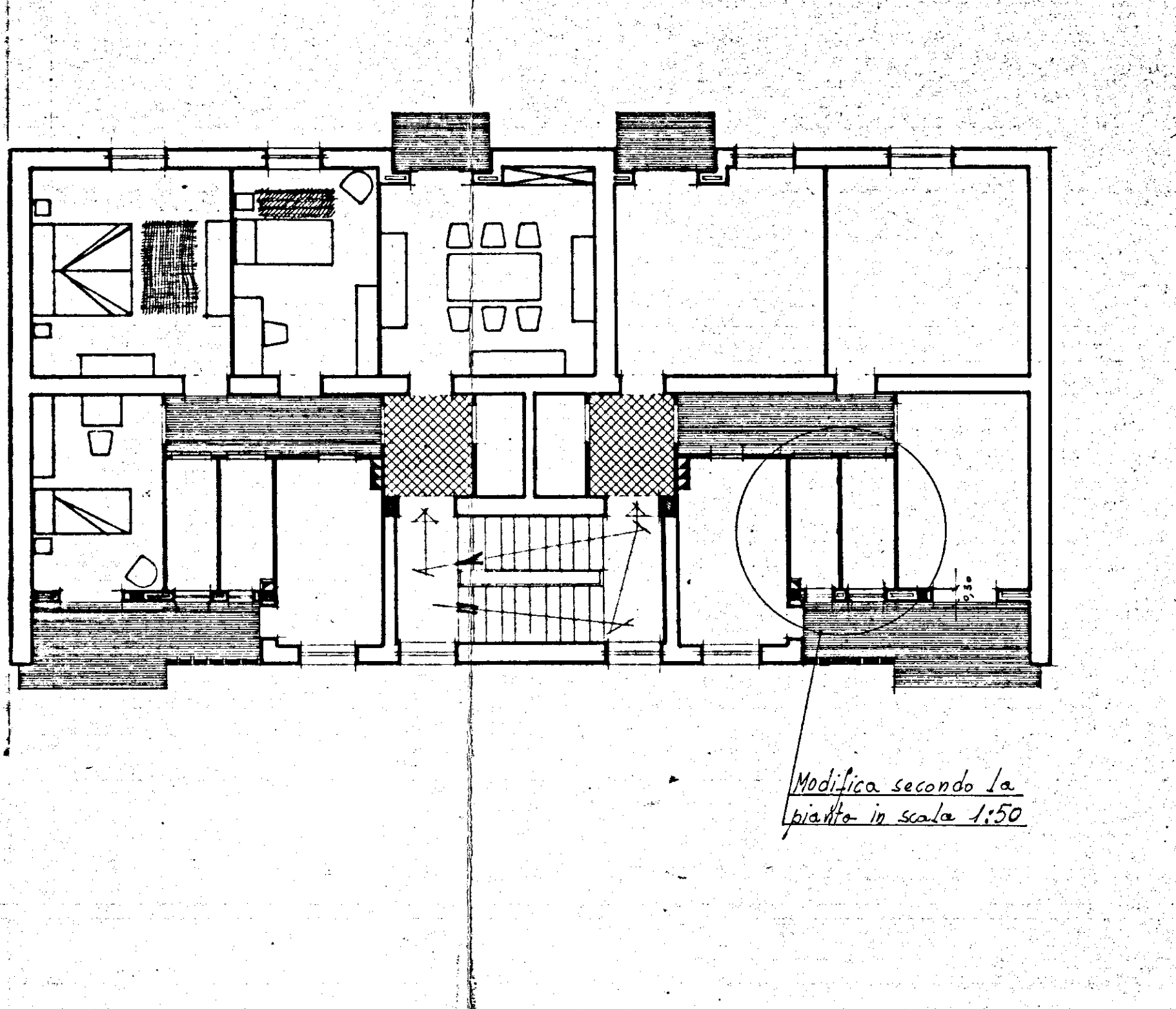
PIANO TIPO
