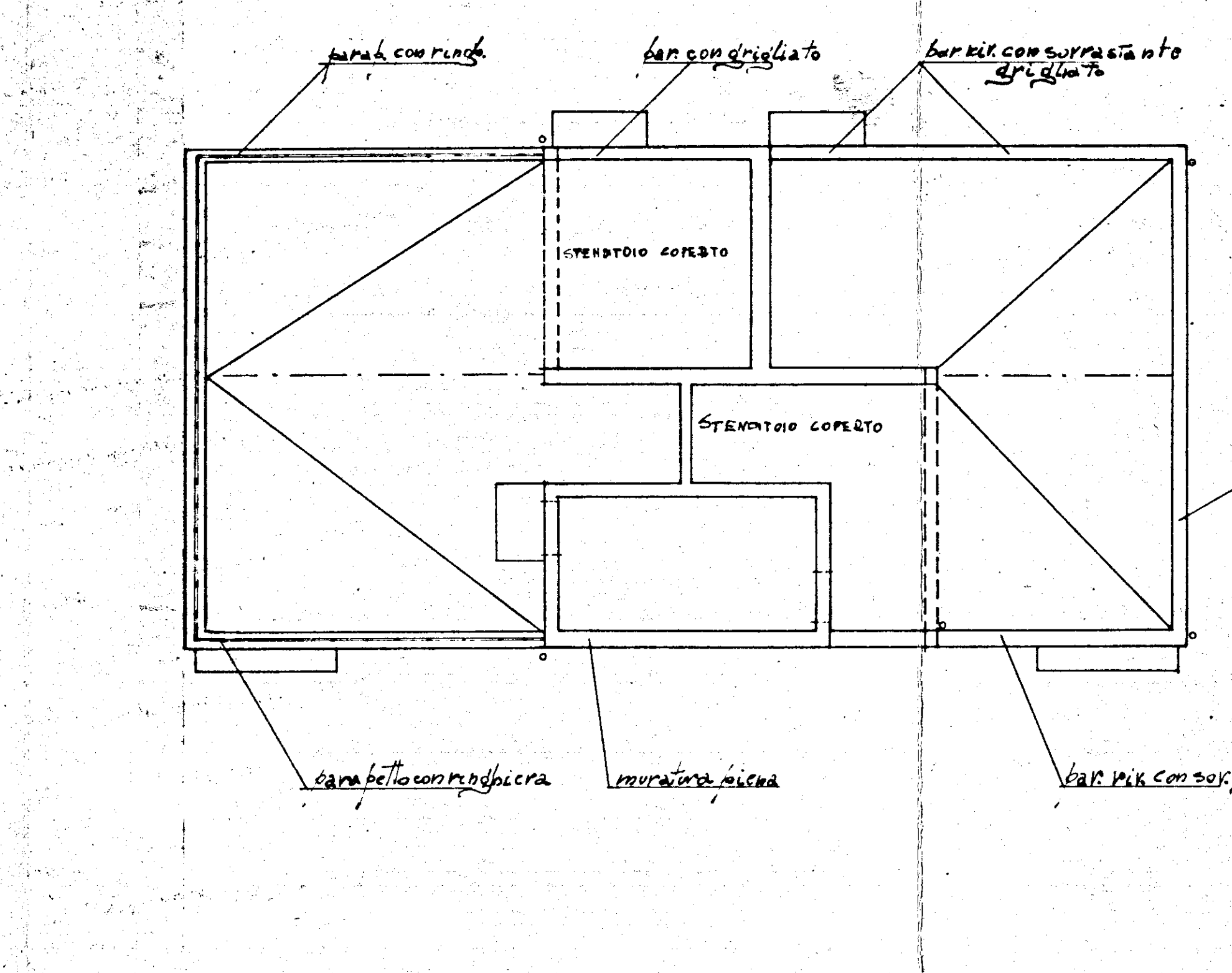
PIANTA TERRAZZA
