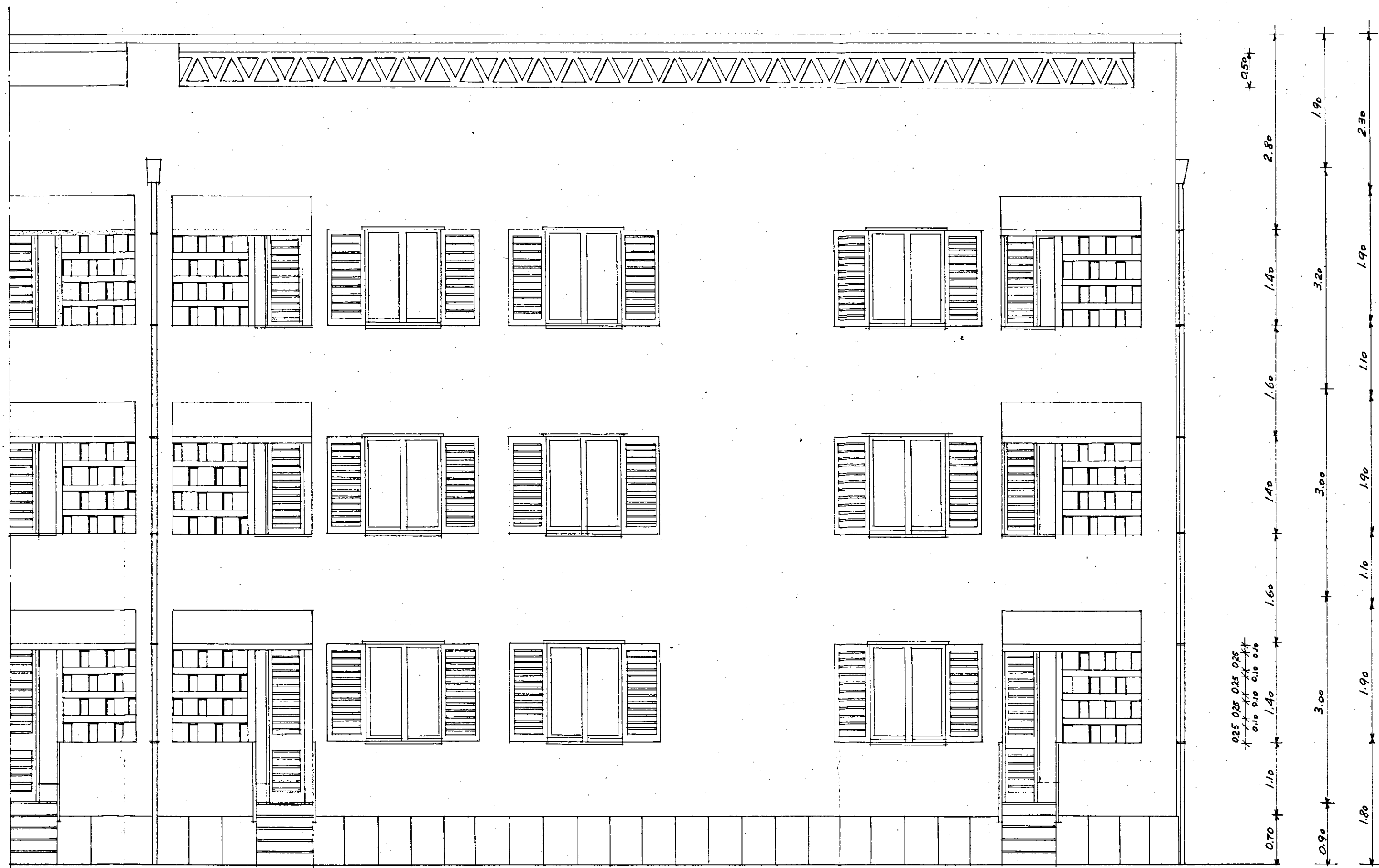
DISEGNO N° 406 PROSPETTO SUD-OVEST (EDIFICIO 1) " NORD-OVEST (EDIFICIO 2) PARTICOLARE DIS. N° 100
