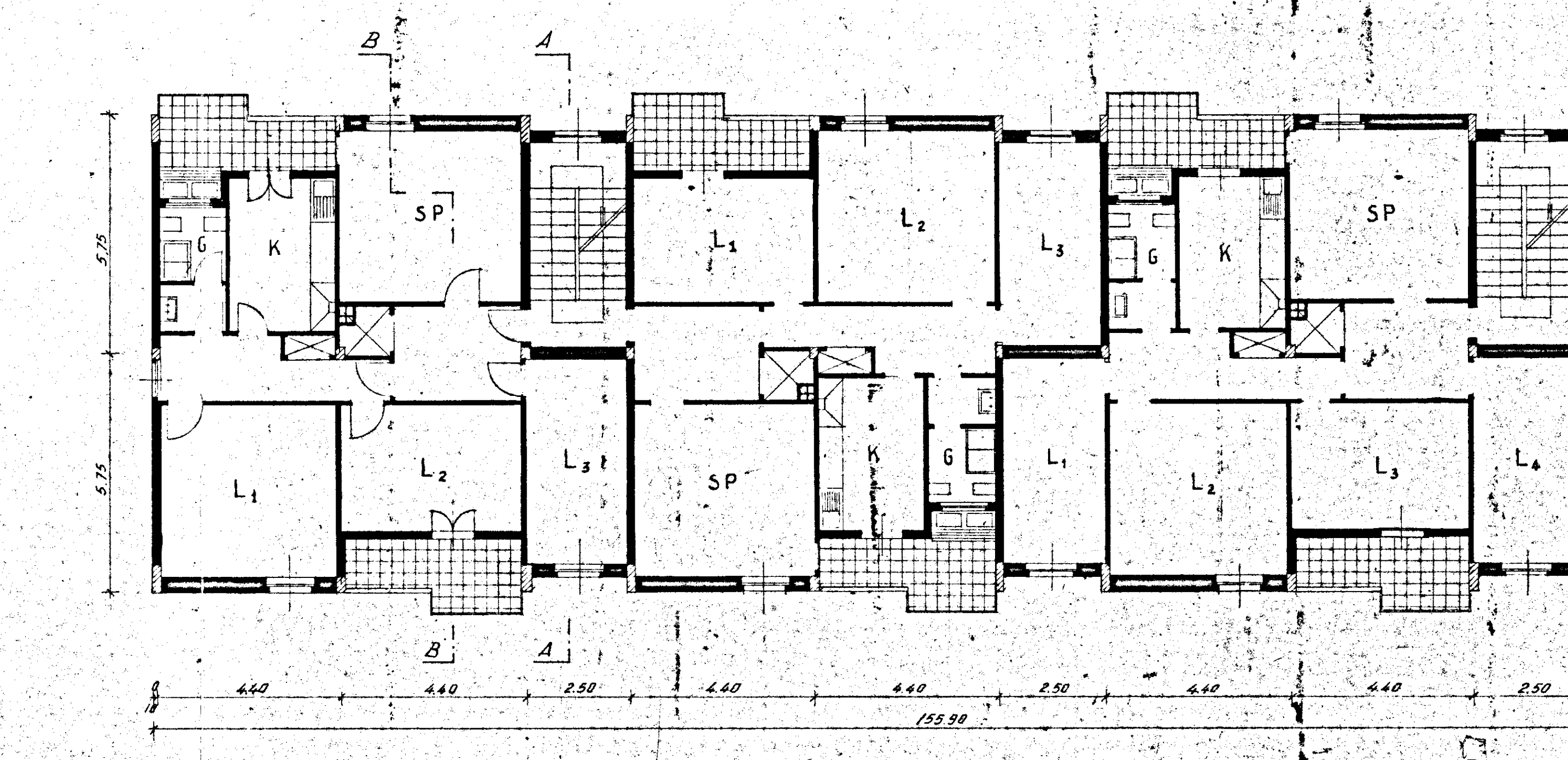
PIANTA DEL PIANO TIPO
