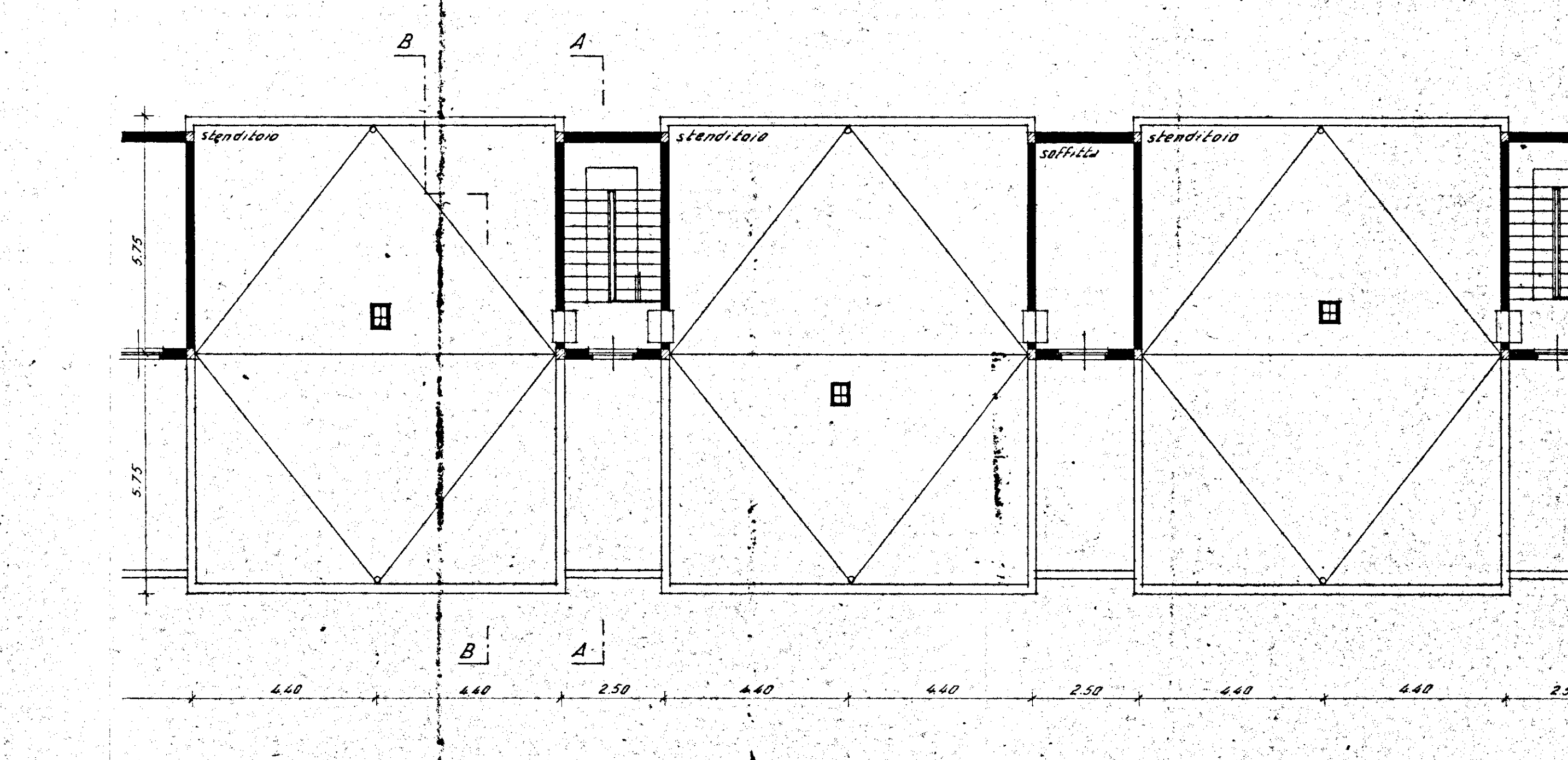
PIANTA DEL PIANO DELLE TERRAZZE DI COPERTURA
