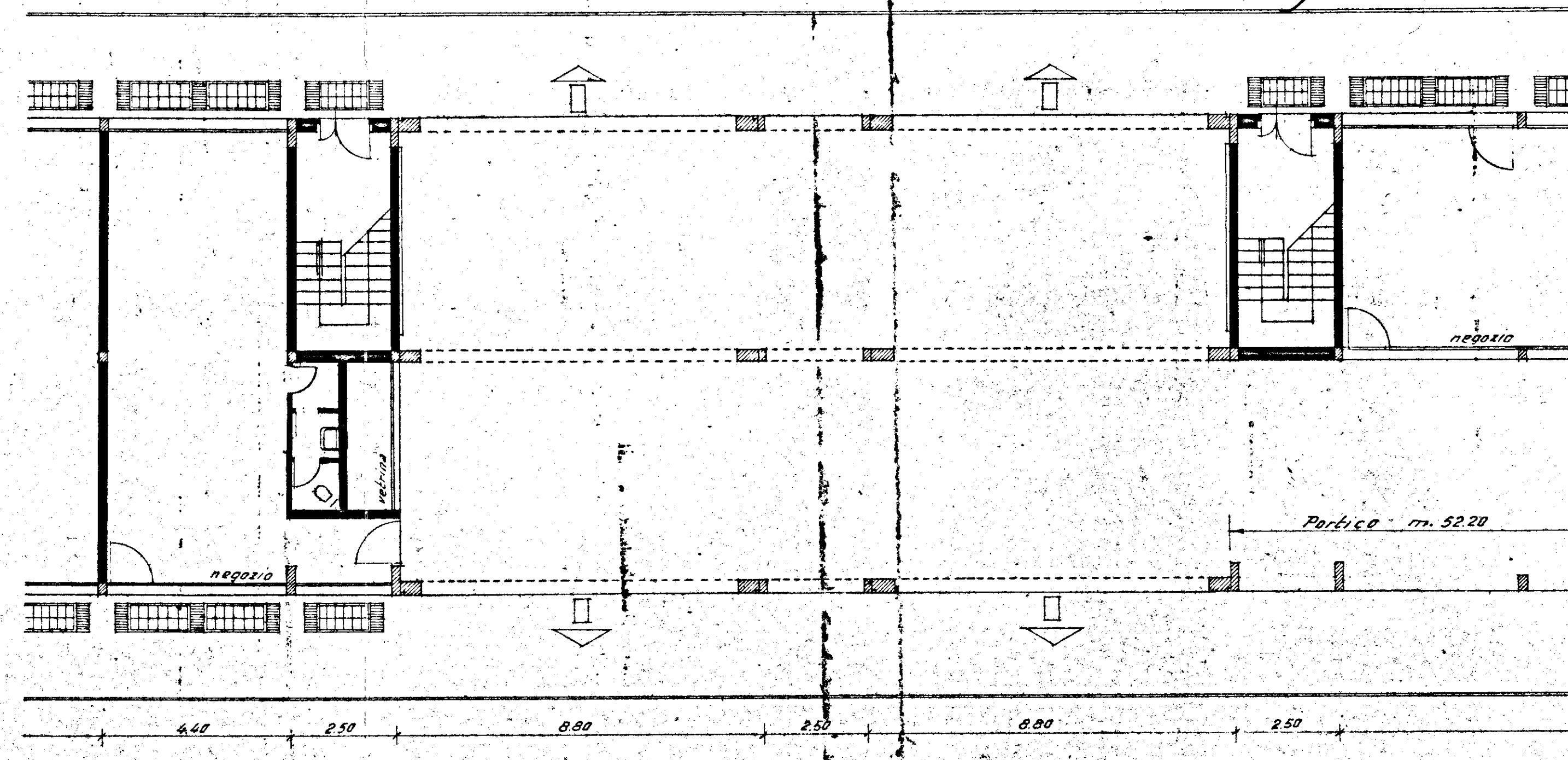
PIANTA DEL PIANO TERRENO IN CORRISPONDENZA DEL PASSAGGIO PEDONALE E INIZIO PORTICO
