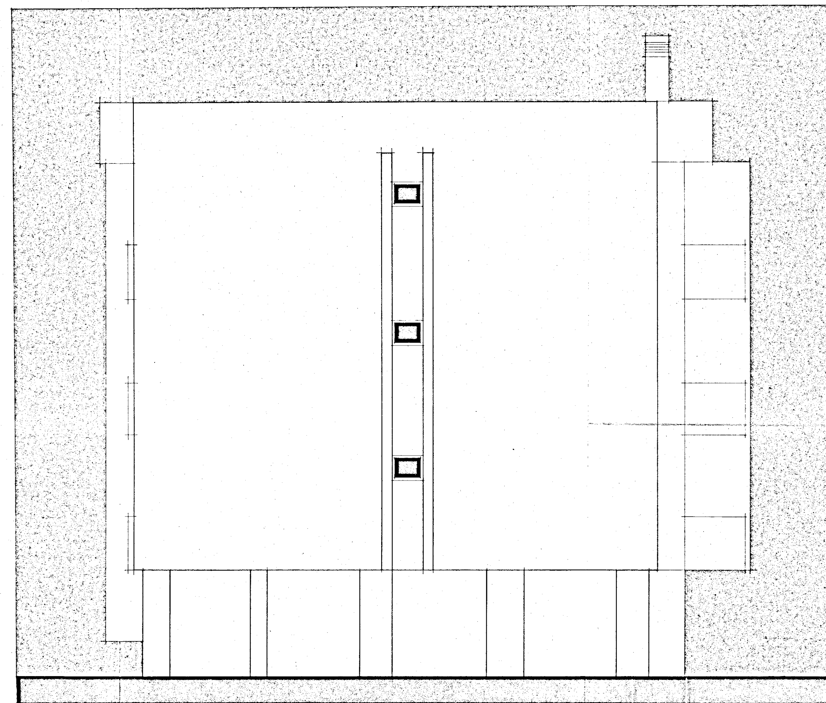
PROSPETTO NORD
