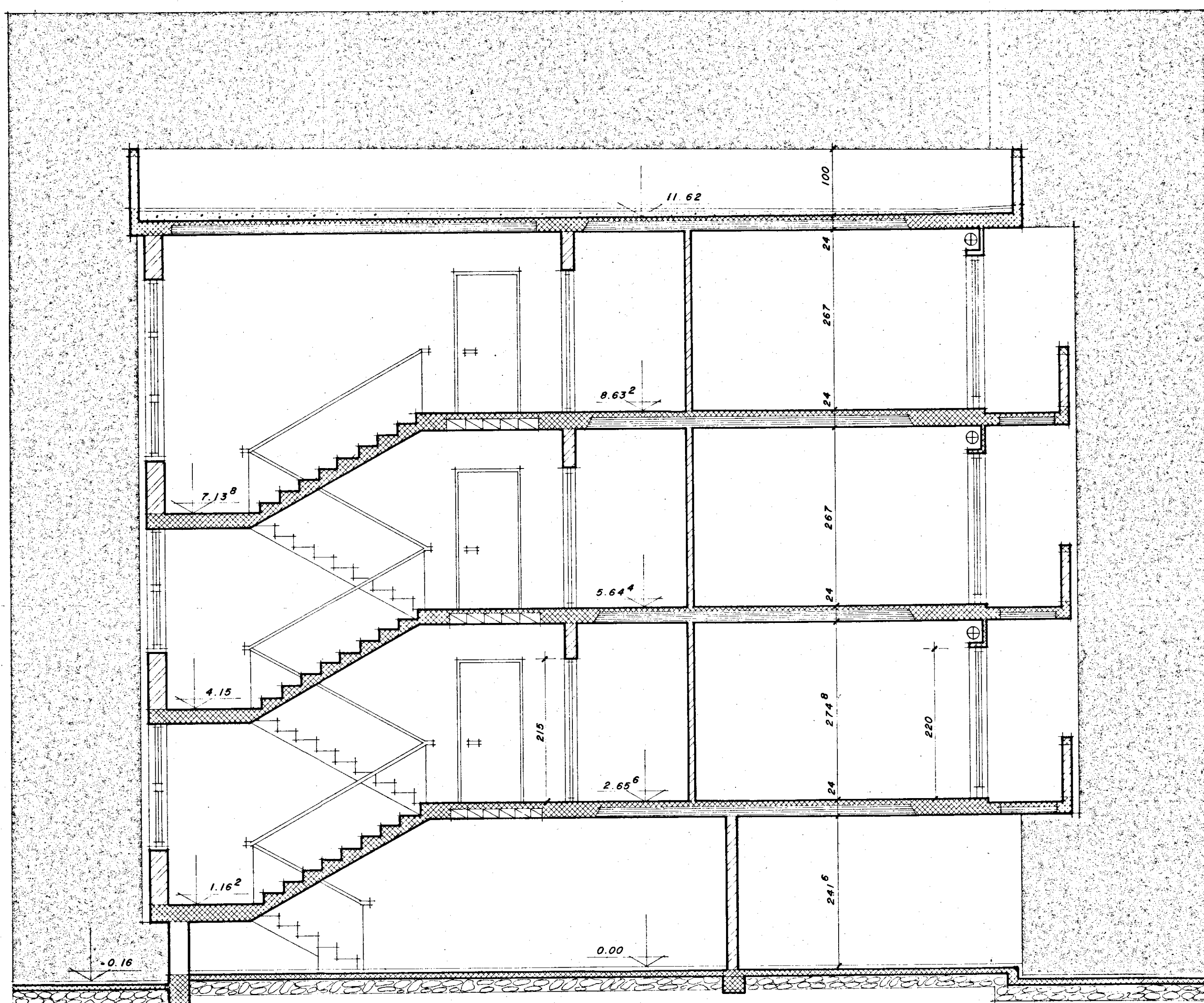
SEZIONE X - X
