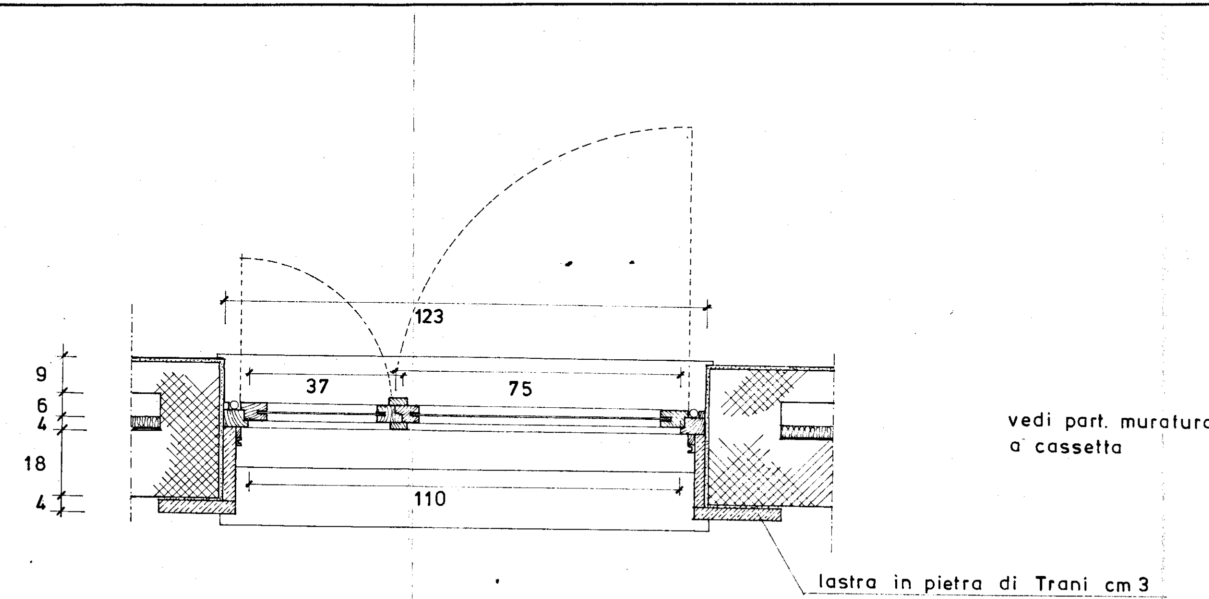
PARTICOLARE ATTACCO INFISSI-MURATURA
