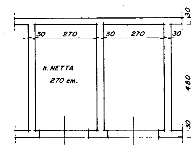
PARTICOLARE BOX ESTERNI RAPP. 1:100
