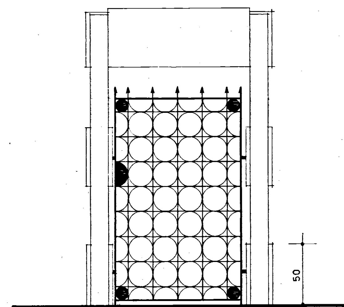
PROSPETTO
