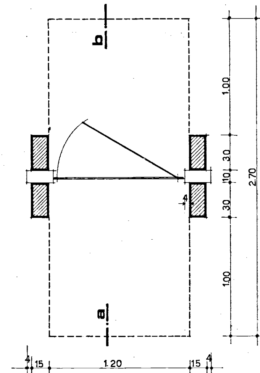
PIANTA
