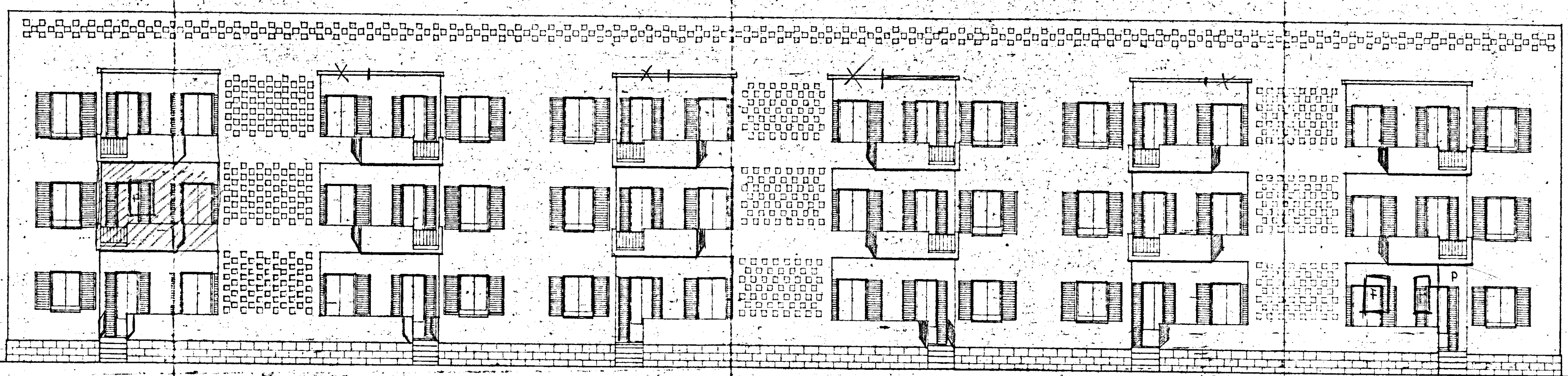
DIS. N° 125 PROSPETTO A SUD-OVEST RAPP. 1:100
