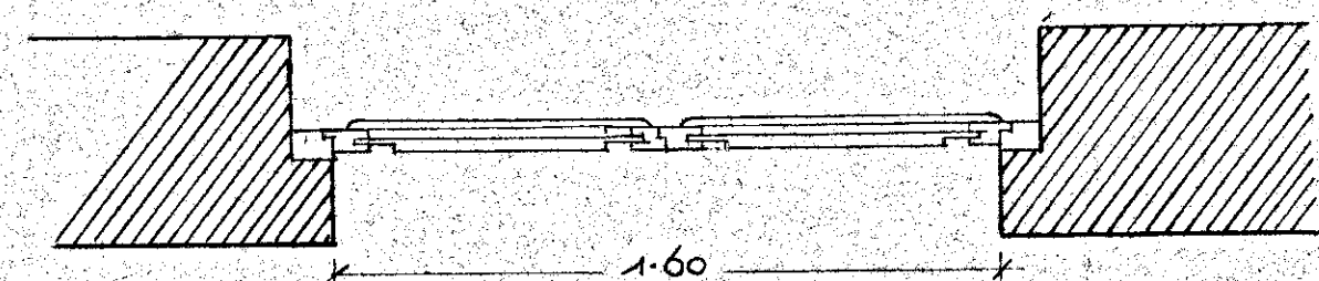
SEZIONE TRASVERSALE
