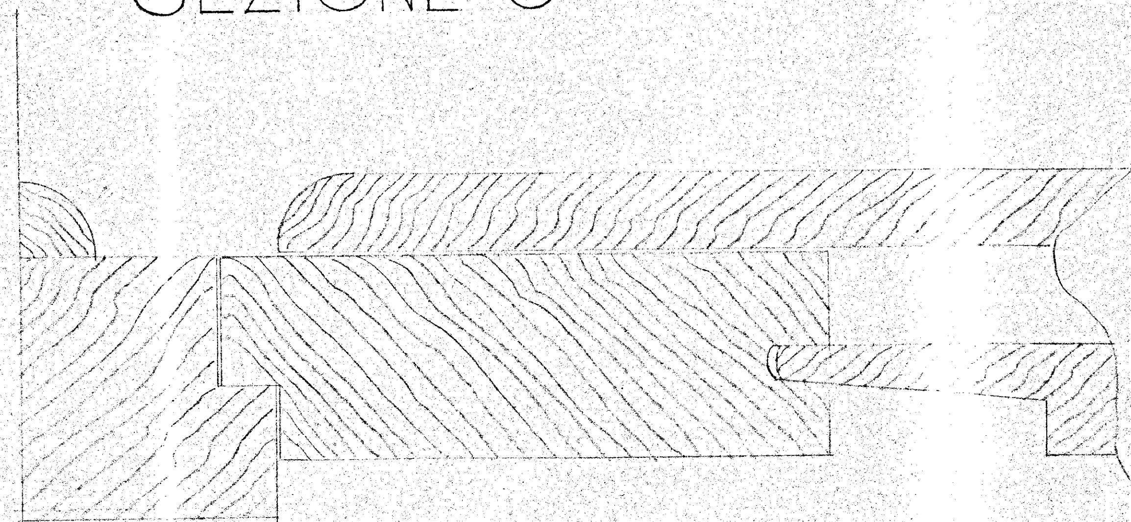
SEZIONE C
