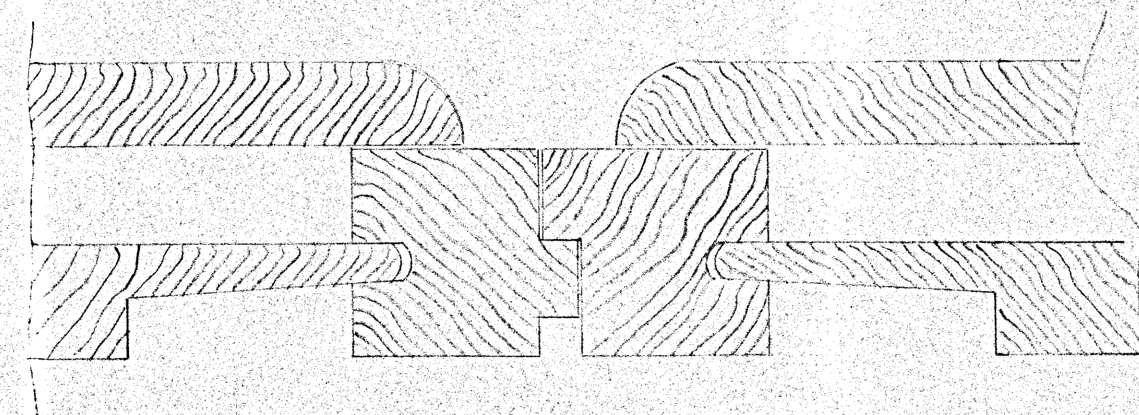
SEZIONE B
