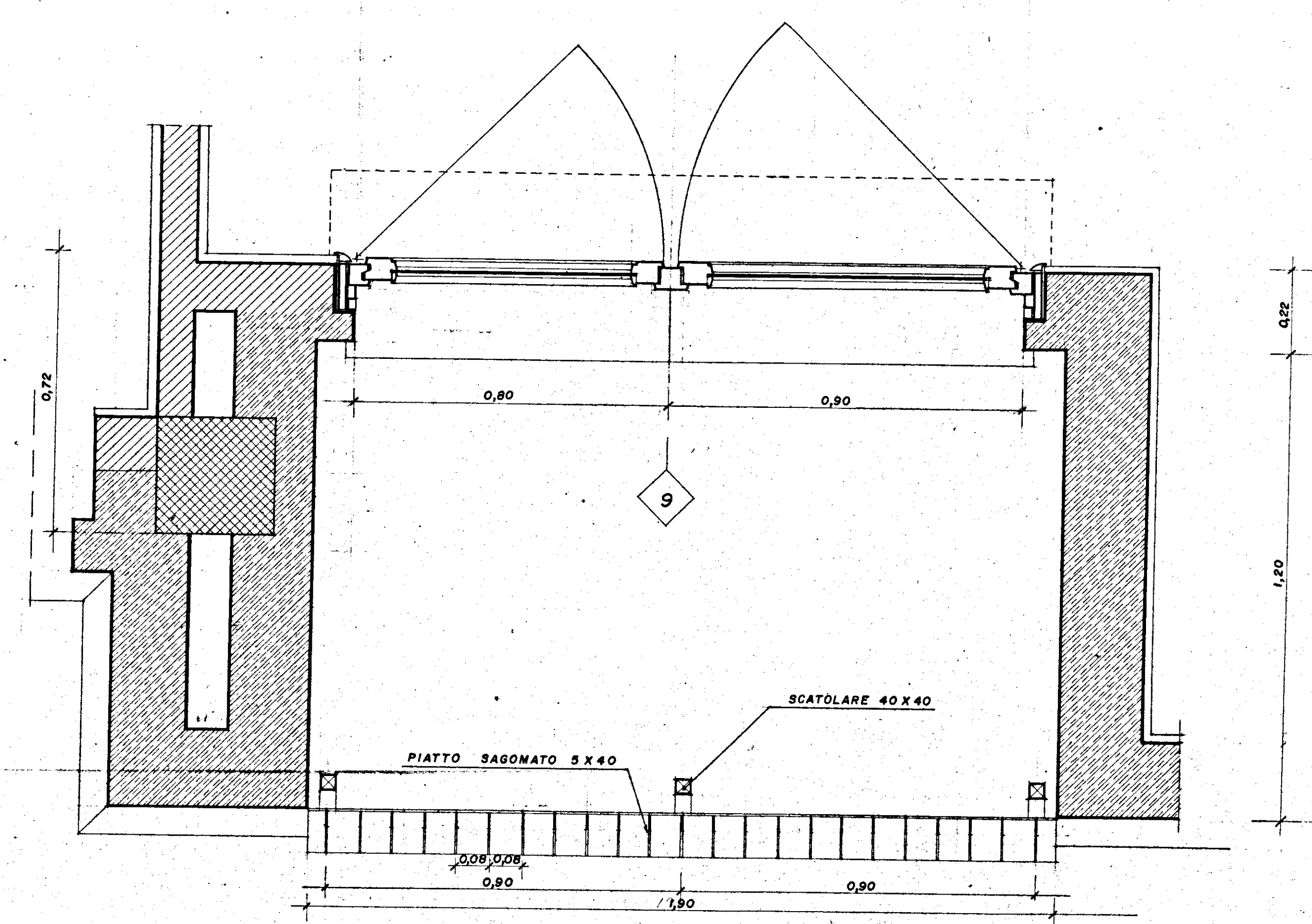
PIANTA
