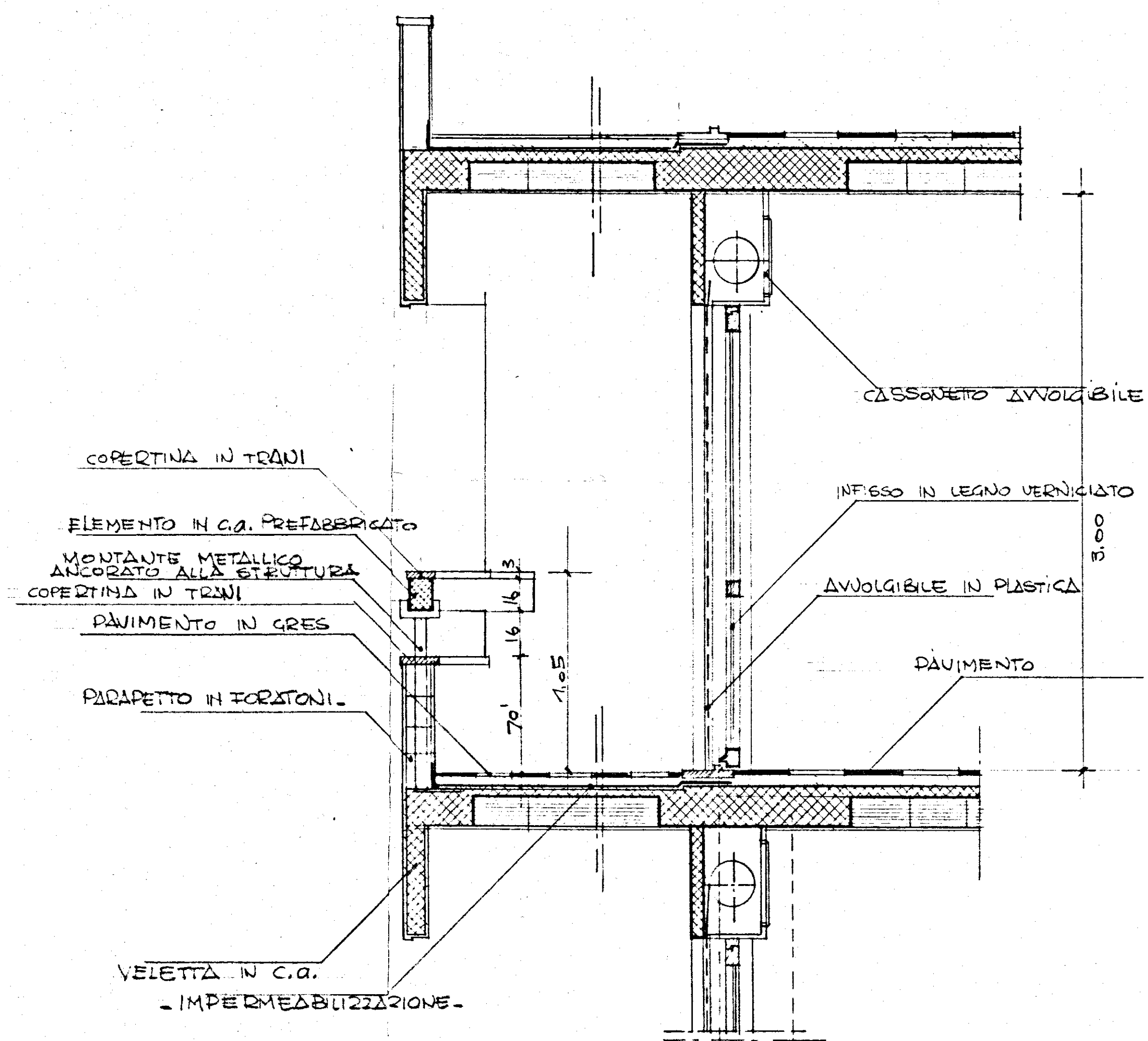
DETTAGLIO SEZIONE BALCONI RAPP. 1:20 -
