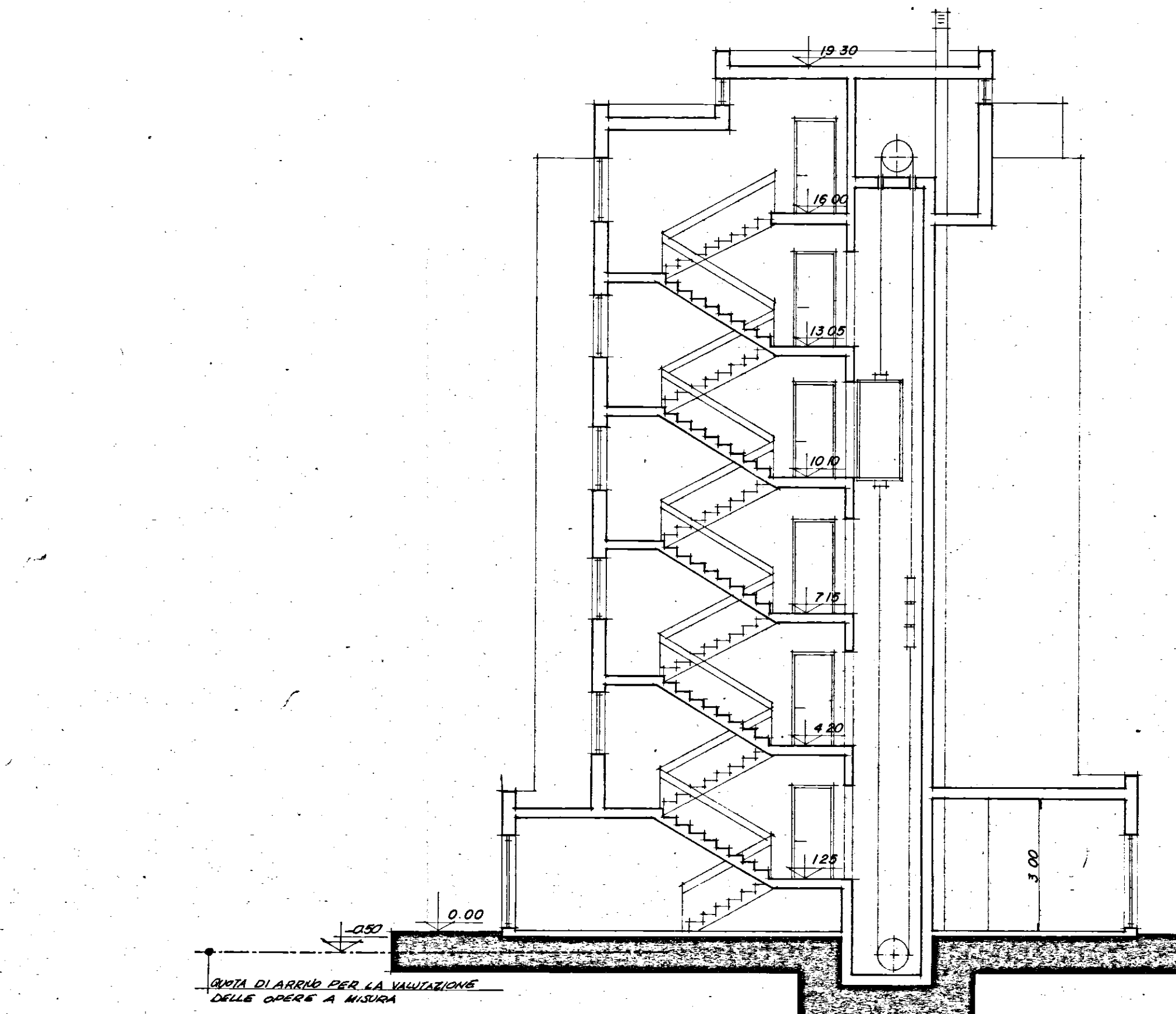
SEZIONE Y - Y
