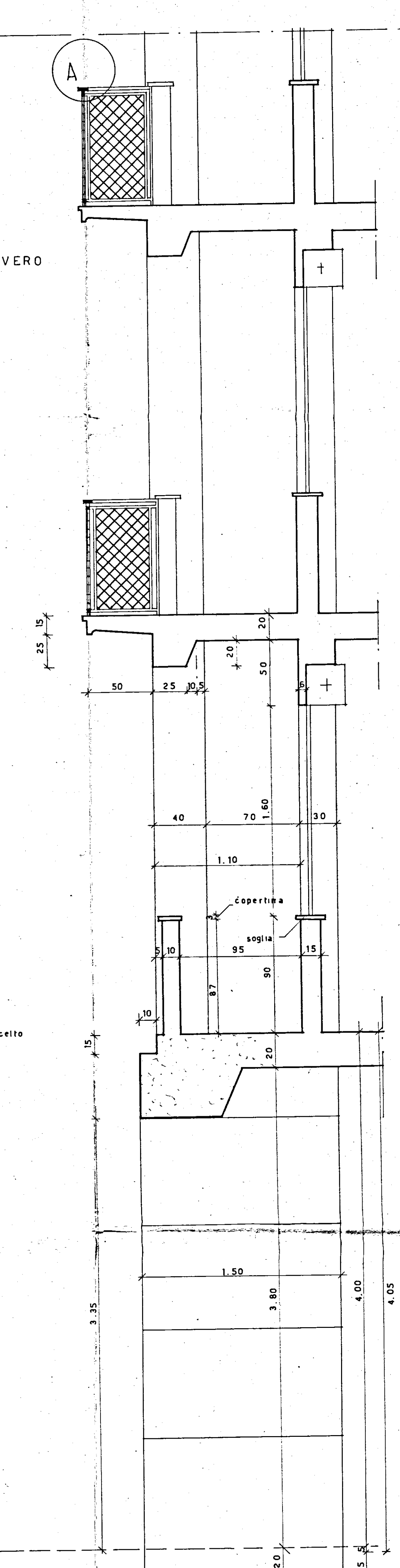
SEZIONE A-B
