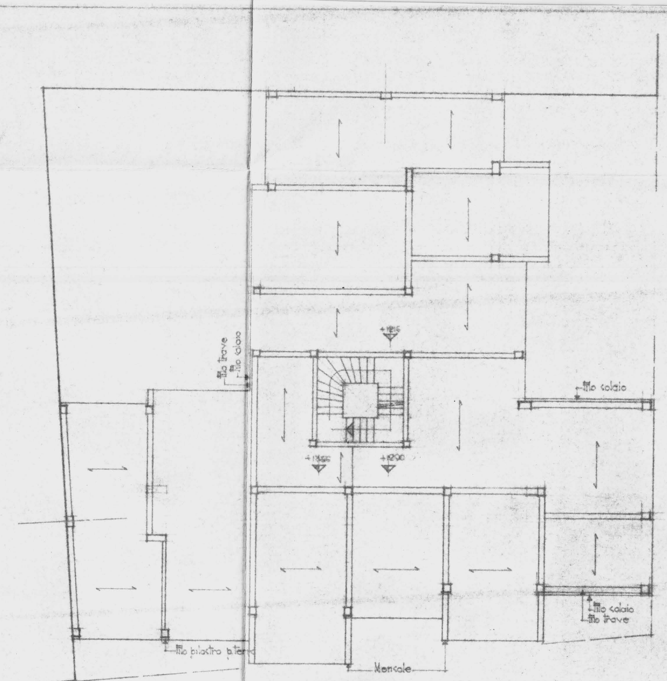
SCHEMA STRUTTURE Scala 1:100
