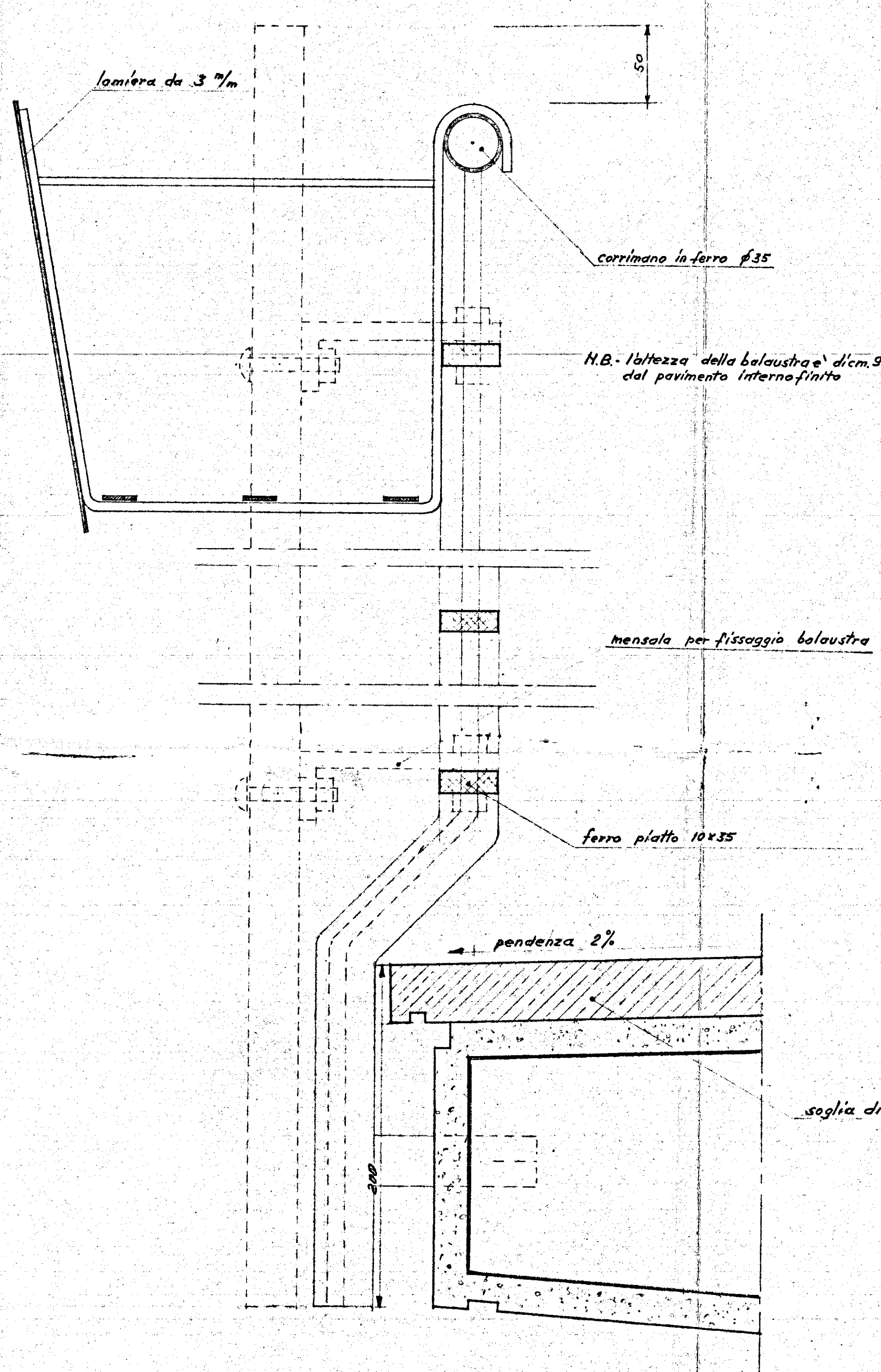
SEZIONE A-A
