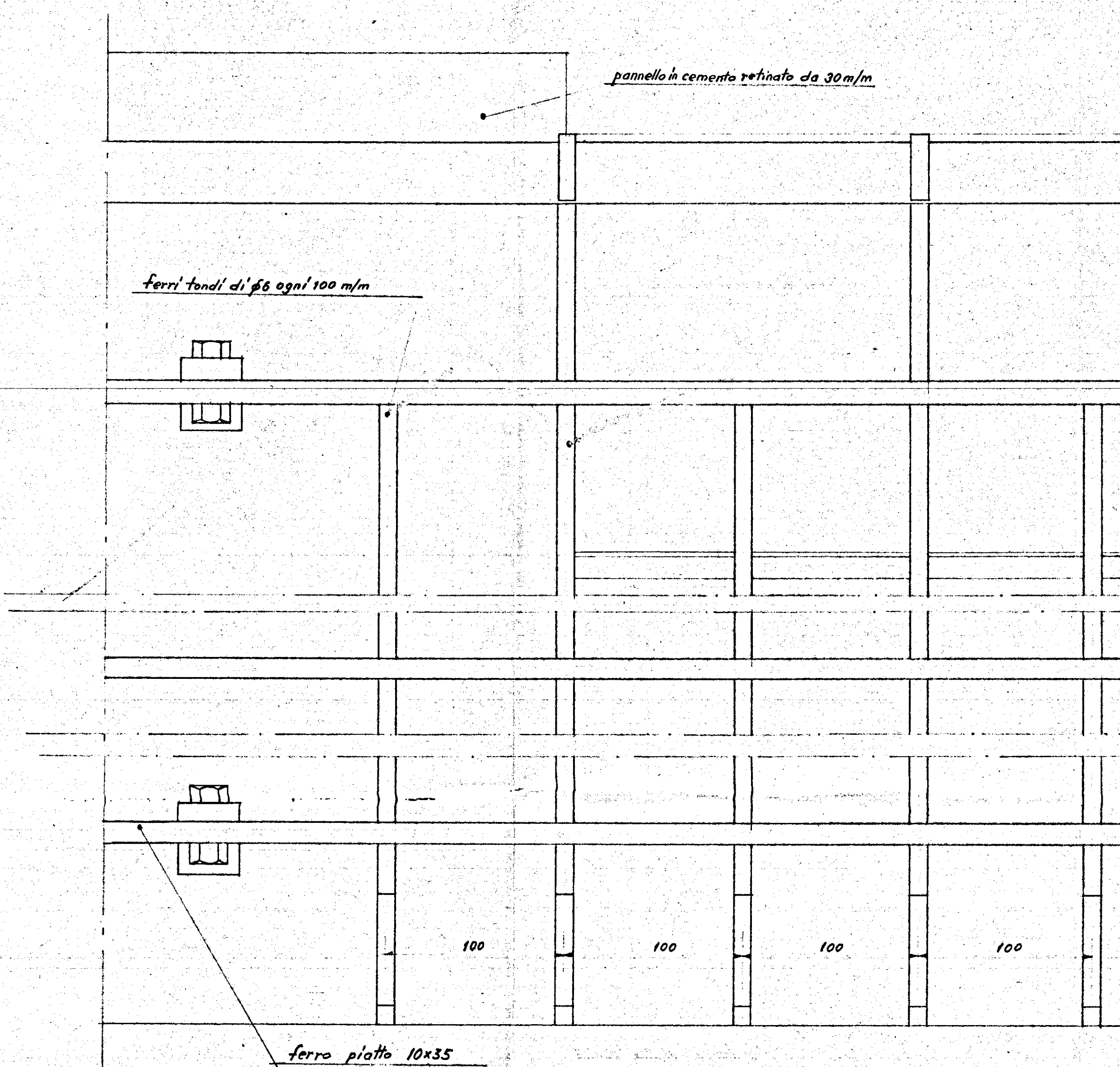
PROSPETTO INTERNO
